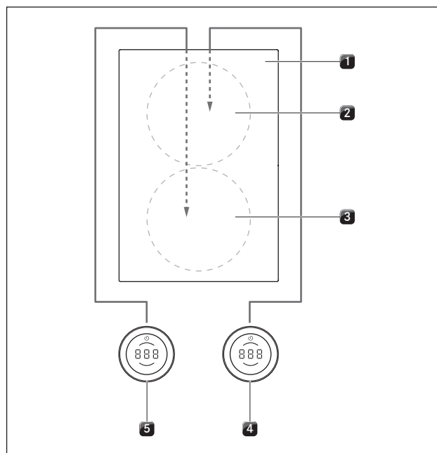
Ilustracja 4.23 Przyłączenie pól grzewczych dla montażu w pozycji obróconej o 180° i urządzeń z przylączami z przodu
