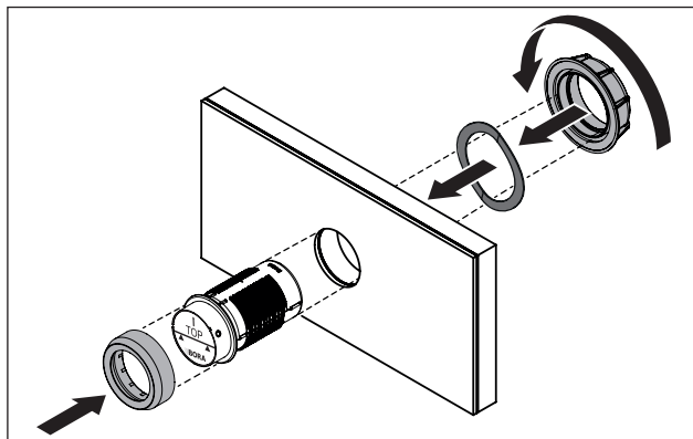
Ilustracja 4.14 Montaż gałki obsługi
