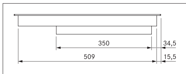
Ilustracja 2.3 Wymiary urządzenia PKCH3 – widok z boku
