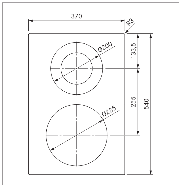
Ilustracja 2.1 Wymiary urządzenia PKCH3 – widok z góry
