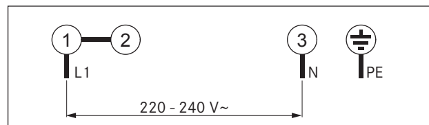
Ilustracja 4.25 Schemat podłączenia 1-fazowy
