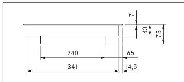
Ilustracja 2.2 Wymiary urządzenia PKCH3 – widok z przodu
