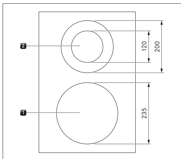
Ilustracja 3.5 Budowa płyty grzewczej PKCH3 i wielkość pól grzewczych
