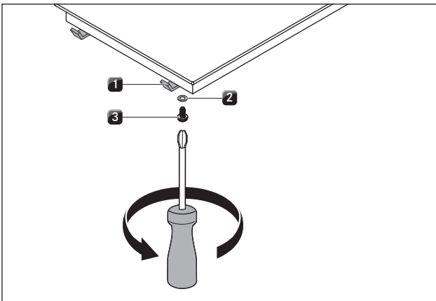
Afb. 5.18 Bevestigingsklemmen
