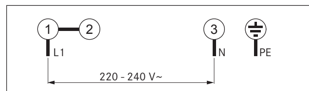
Afb. 5.25 Aansluitschema 1-fasig
