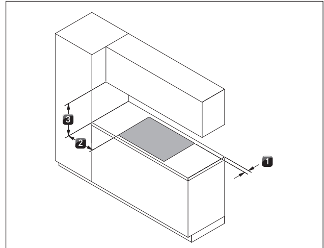
Afb. 5.19 Minimumafstanden bij 180° gedraaide inbouw
