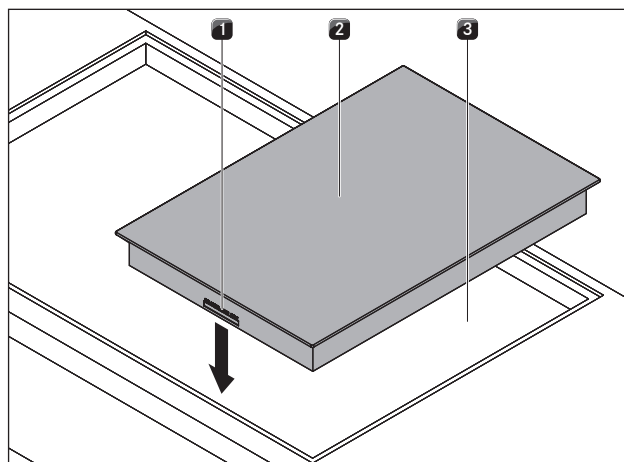
Afb. 5.16 Kookveld plaatsen
