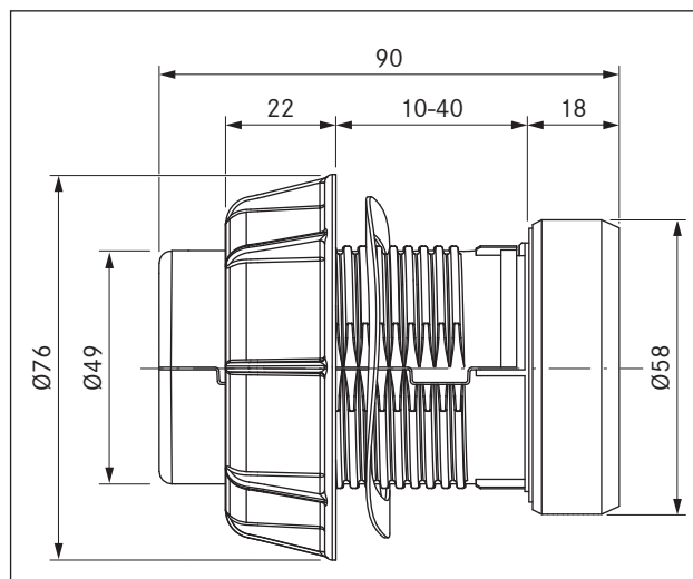
bild 3.8 Apparatmått vridknapp
