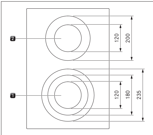
bild 4.5 Konstruktion spishäll PKC3 och storleken på kokzonerna
