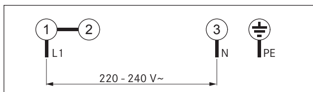
bild 5.25 Kopplingsschema 1-fasigt
