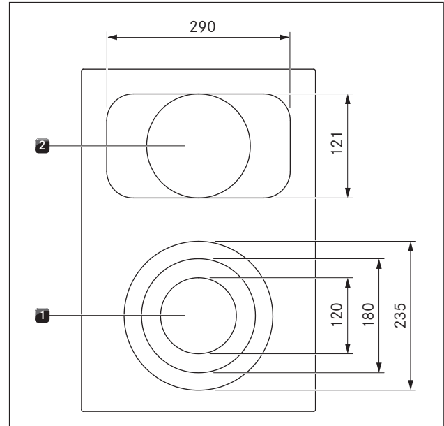
bild 4.6 Konstruktion spishäll PKCB3 och storleken på kokzonerna
