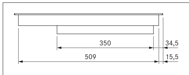
bild 3.6 PKCB3 apparatmått bild från sidan
