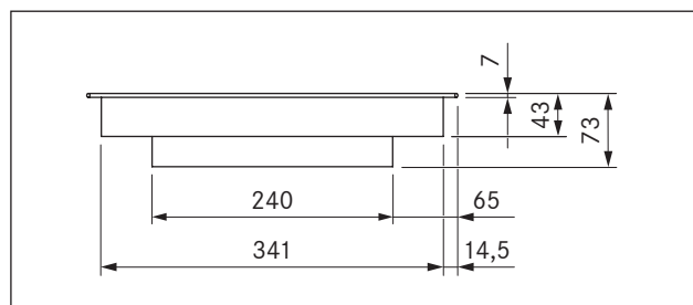
bild 3.5 PKCB3 apparatmått bild framifrån
