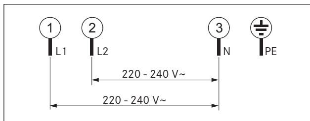
bild 5.26 Kopplingsschema 2-fasigt
