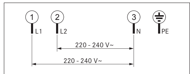
Afb. 5.26 Aansluitschema 2-fasig
