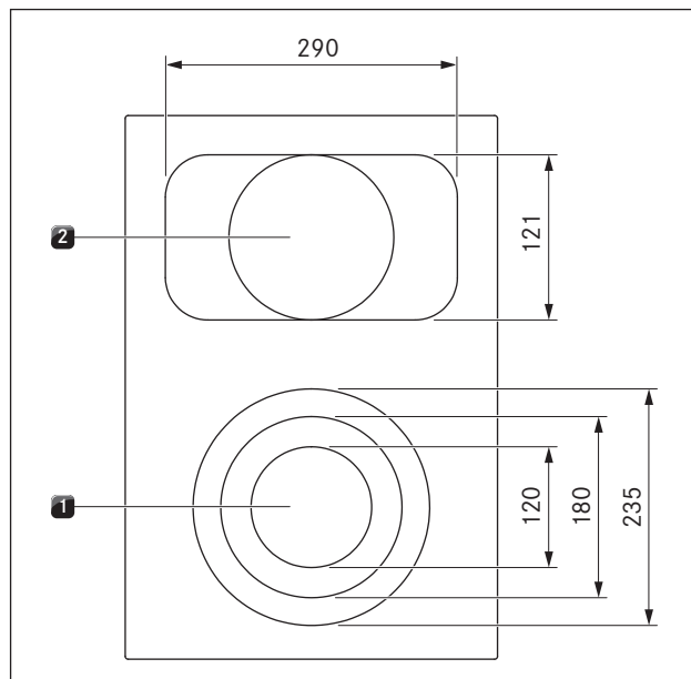
Afb. 4.6 Opbouw kookveld PKCB3 en grootte van de kookzones
