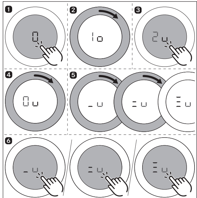
Afb. 6.10 Warmhoudfunctie activeren (PKC3, PKCB3, PKCH3)
