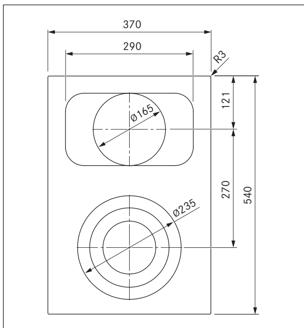
Afb. 3.4 PKCB3 toestelafmetingen bovenaanzicht
