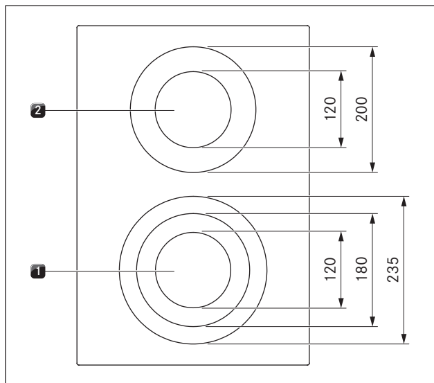
Afb. 4.5 Opbouw kookveld PKC3 en grootte van de kookzones
