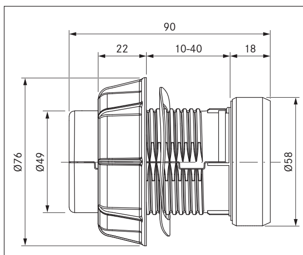
Afb. 3.8 Toestelafmetingen bedieningsknop
