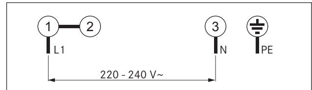
Afb. 5.25 Aansluitschema 1-fasig
