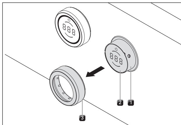
Afb. 7.1 Knopring verwijderen
