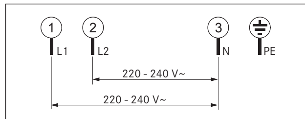
Fig. 5.26 Schema di collegamento bifase
