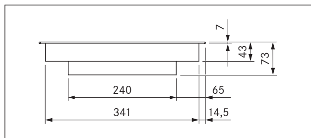
Fig. 3.5 PKCB3 dimensioni apparecchio vista frontale
