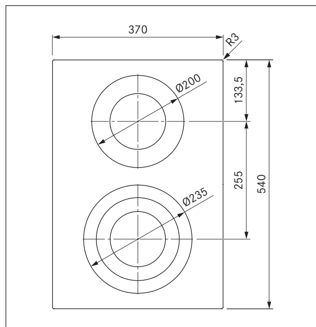
Fig. 3.1 PKC3 dimensioni apparecchio vista dall'alto
