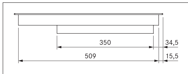
Fig. 3.6 PKCB3 dimensioni apparecchio vista laterale
