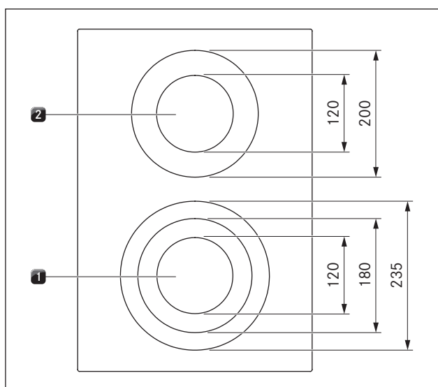
Fig. 4.5 Montaggio piano cottura PKC3 e dimensioni delle zone cottura
