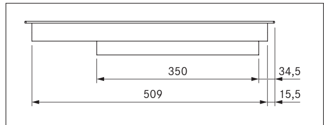
Abb. 3.3 PKC3 Gerätemaße Seitenansicht
