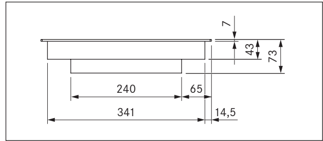
Abb. 3.2 PKC3 Gerätemaße Vorderansicht
