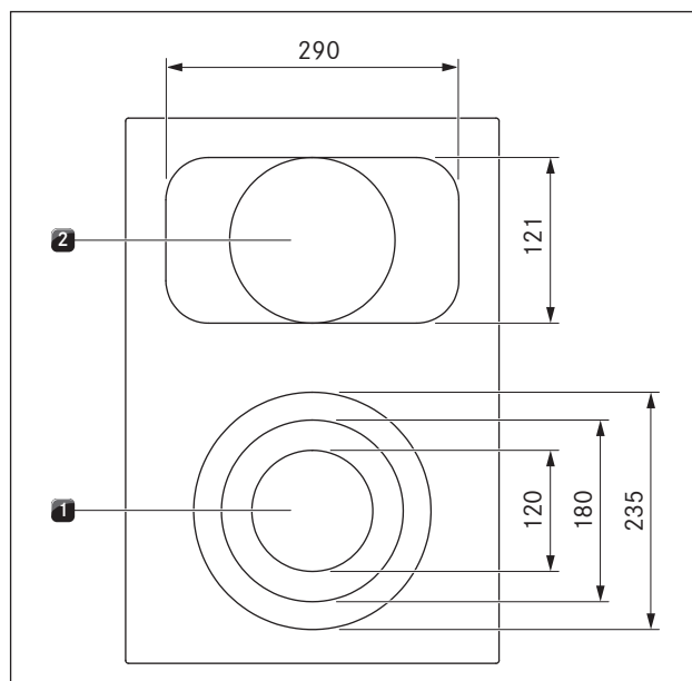
Abb. 4.6 Aufbau Kochfeld PKCB3 und Größe der Kochzonen
