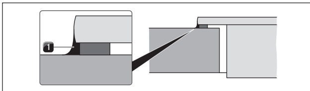
Abb. 5.28 Silikondichtmasse bei Aufsatzmontage
