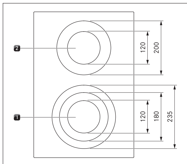
Abb. 4.5 Aufbau Kochfeld PKC3 und Größe der Kochzonen
