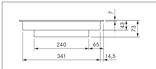
Obr. 3.2 Rozměry produktu PKC3 – pohled zepředu
