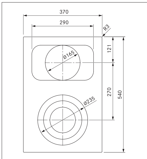
Obr. 3.4 Rozměry produktu PKCB3 – pohled shora
