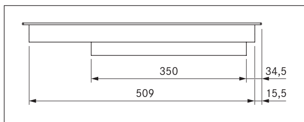
Obr. 3.3 Rozměry produktu PKC3 – pohled z boku
