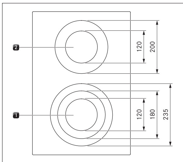
Obr. 4.5 Konstrukce varné desky PKC3 a rozměry varných zón
