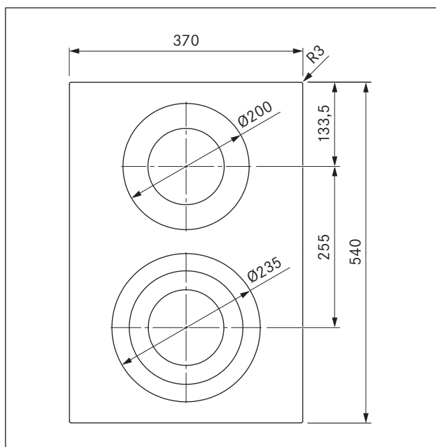
Obr. 3.1 Rozměry produktu PKC3 – pohled shora
