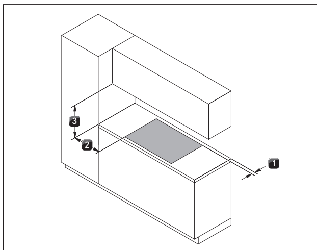
Obr. 5.1 Minimální vzdálenosti
