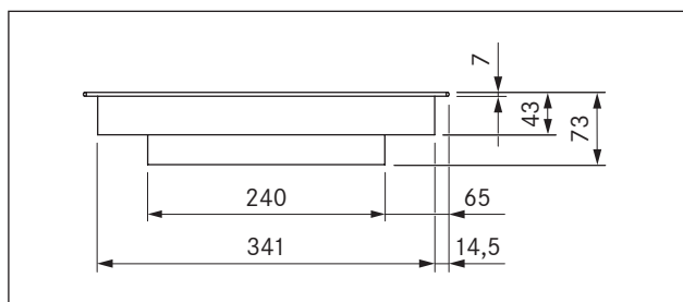
Obr. 3.5 Rozměry produktu PKCB3 – pohled zepředu
