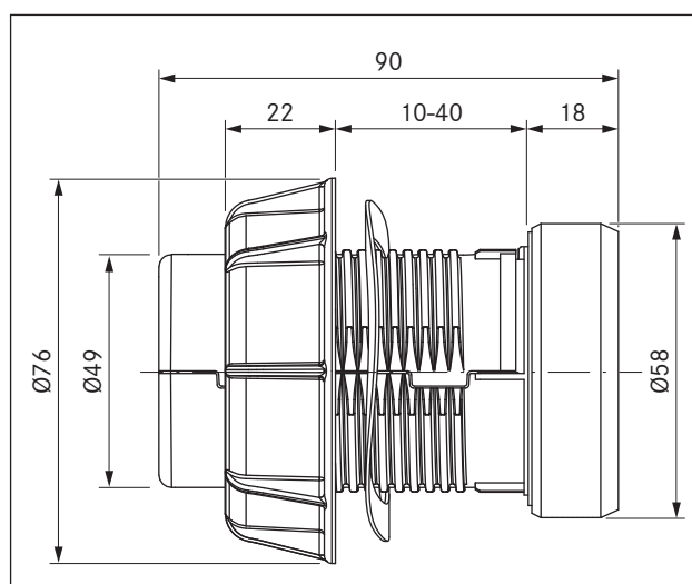
Obr. 3.8 Rozměry ovládacího kolečka
