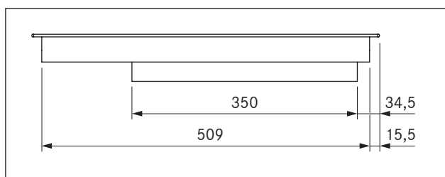
Obr. 3.6 Rozměry produktu PKCB3 – pohled z boku
