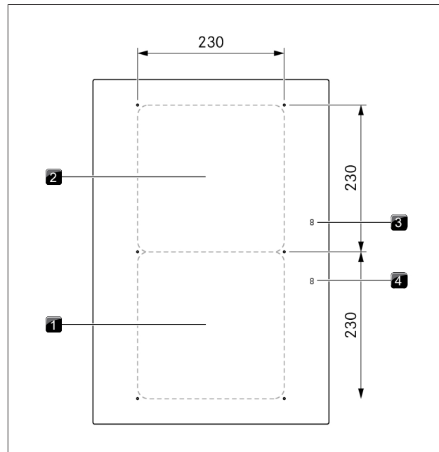
Fig. 3.8 Montaggio piano cottura PKFI3 e dimensioni delle zone cottura
