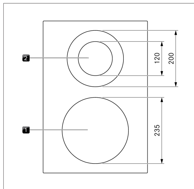
Fig. 3.13 Montaggio piano cottura PKCH3 e dimensioni delle zone cottura
