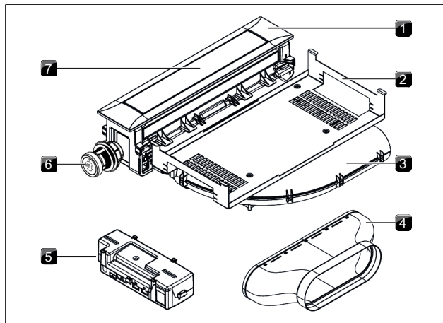
Fig. 3.5 Aspiratore per piano cottura PKA3/PKA3AB
