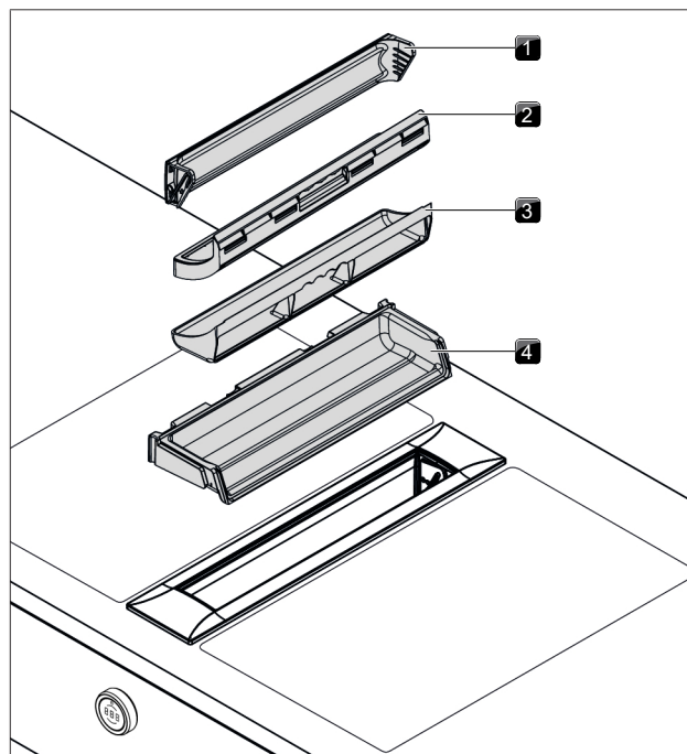
Fig. 3.7 Componenti filtro
