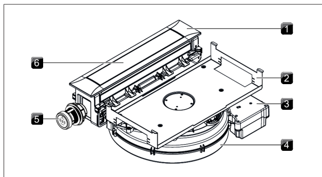
Fig. 3.6 Sistema di aspirazione per piano cottura PKAS3/PKAS3AB
