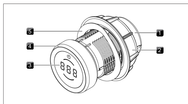
Fig. 3.1 Struttura manopola di comando
