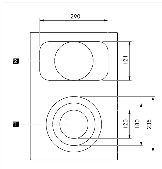
Fig. 3.12 Montaggio piano cottura PKCB3 e dimensioni delle zone cottura
