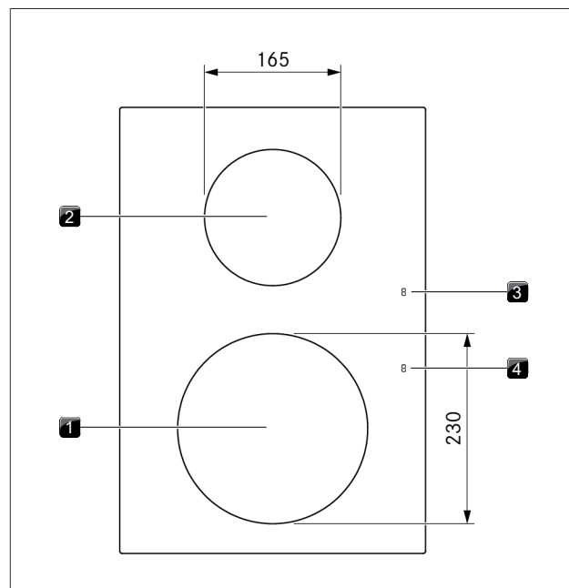
Fig. 3.9 Montaggio piano cottura PKI3 e dimensioni delle zone cottura
