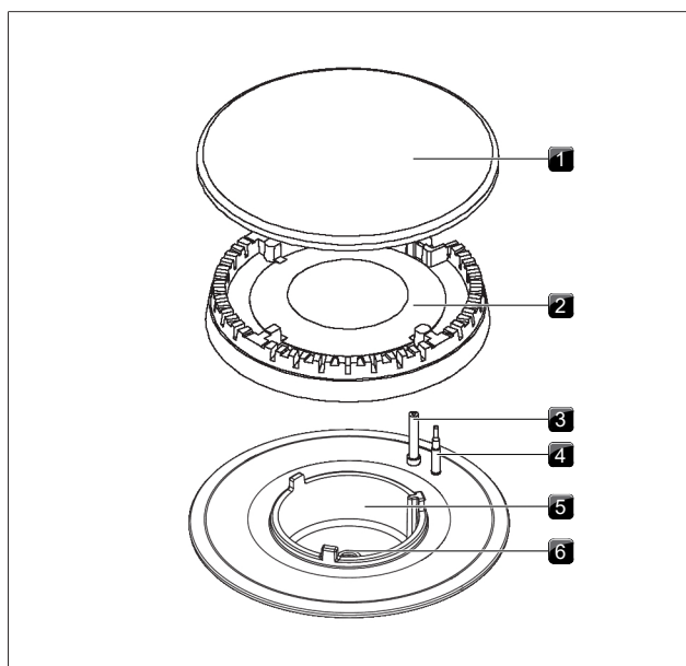
Rys. 7.7 Budowa palnika gazowego
