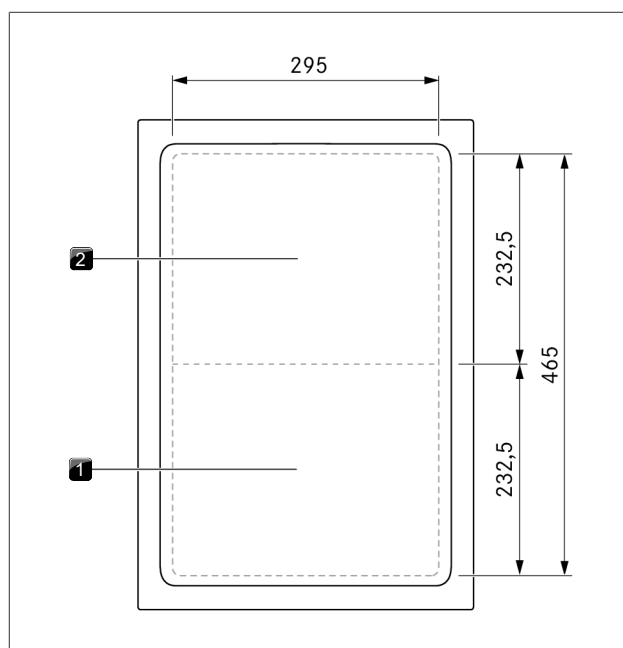
Rys. 3.14 Budowa grilla Tapan ze stali szlachetnej PKT3 i wielkość pól grzewczych
