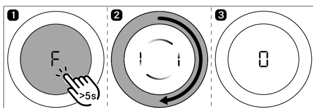
Rys. 5.23 Resetowanie wskaźnika zużycia filtra
