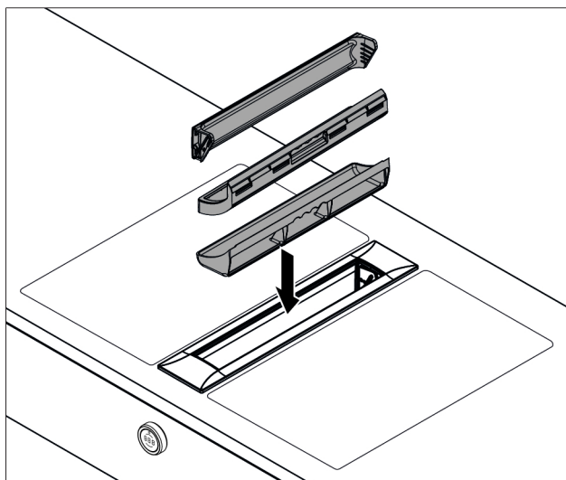
Rys. 7.2 Montaż komponentów
