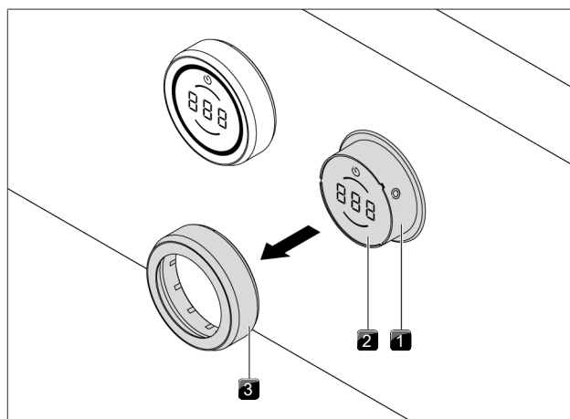
Rys. 7.8 Zdejmowanie pierścienia gałki obsługi
