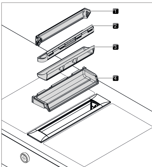
Rys. 3.7 Komponenty filtra
