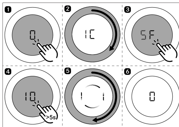
Rys. 5.21 Przedwczesne resetowanie wskaźnika zużycia filtra
