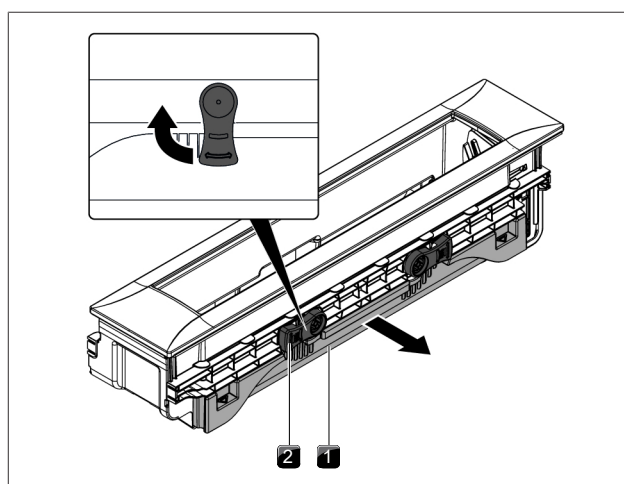
Rys. 7.4 Demontaż wanienki konserwacyjnej
