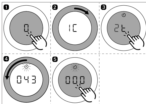
Rys. 5.14 Przedwczesna dezaktywacja minutnika
