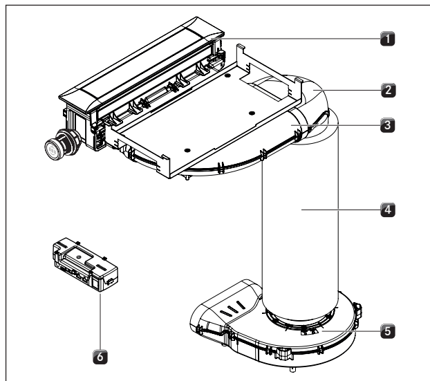
Fig. 4.38 Standardopbygning PKA3/PKA3AB
