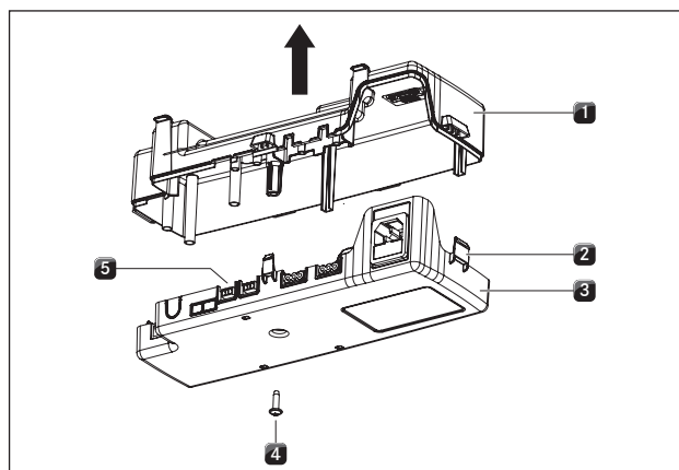
Fig. 4.40 Åbn dækslet på styreenheden
