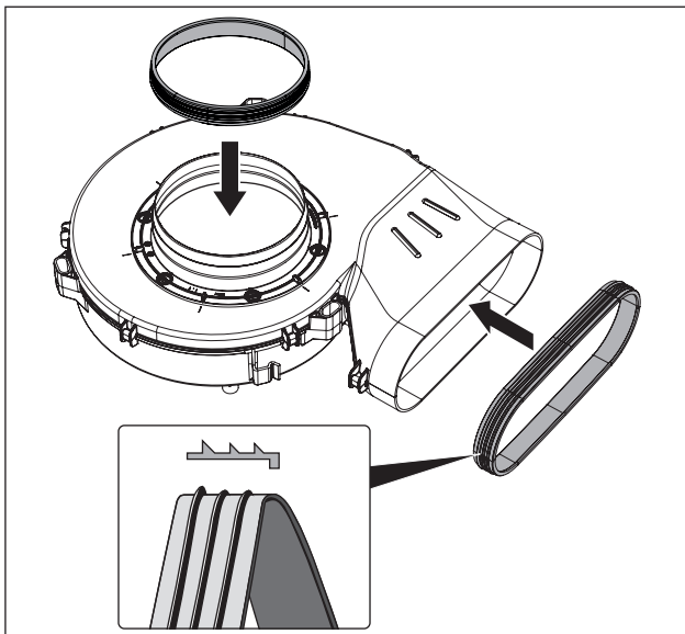
Fig. 4.37 Placer tætningerne på sokkelventilatorens indsugnings- og udsugningsstuds.
