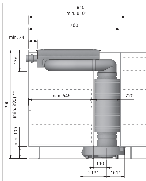
Fig. 4.5 Indbygningsmål for apparater PKA3/PKA3AB med rund lydæmper USDR50 ved standardopbygning
