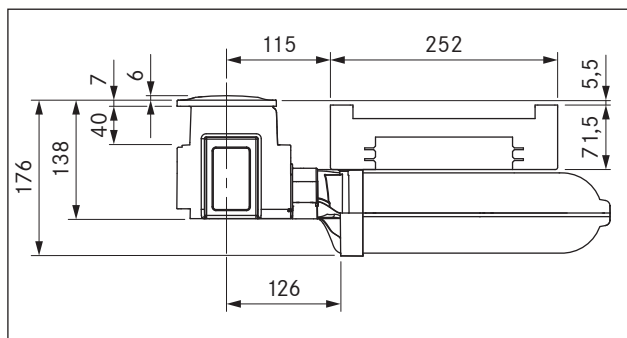
Fig. 3.2 PKA3/PKA3AB apparatmål set forfra
