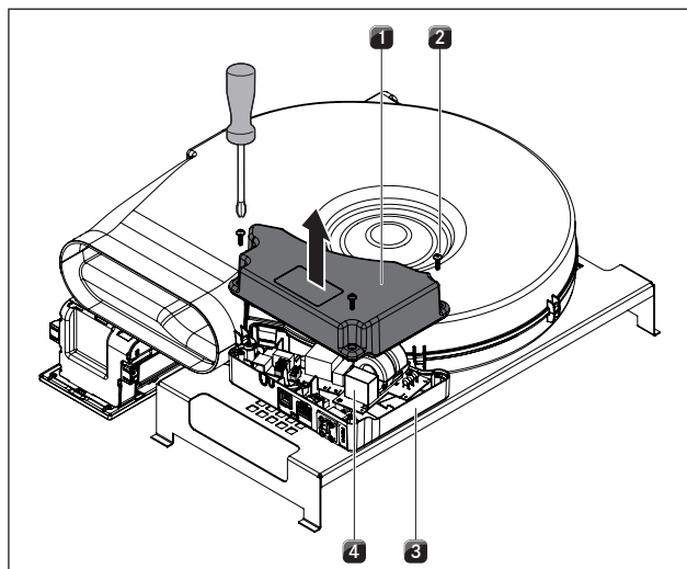
Fig. 4.39 Åbn dækslet på styreenheden
