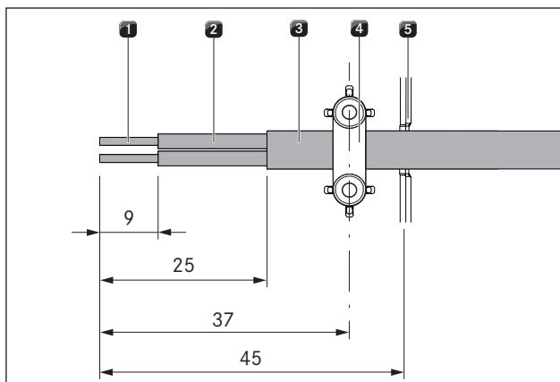
Fig. 4.41 Afisoleringslængder og monteringsposition for tilslutningskablet PKA3/PKA3AB
