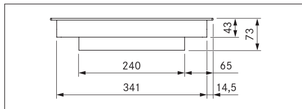
SI. 3.3 Dimenzije naprave PKCH2, pogled od spredaj
