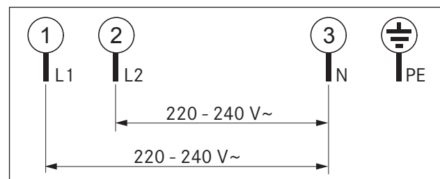
Fig. 5.22 Esquema de ligação bifásica
