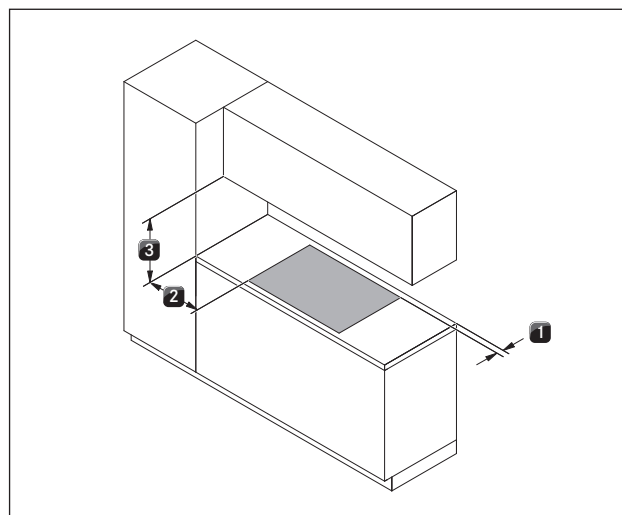
Fig. 5.1 Distância mínima
