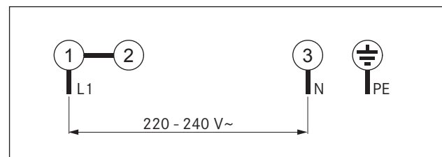
Fig. 5.23 Esquema de ligação monofásica
