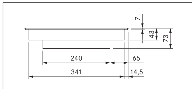
Fig. 3.3 PKCH2 apparatmål visning forfra
