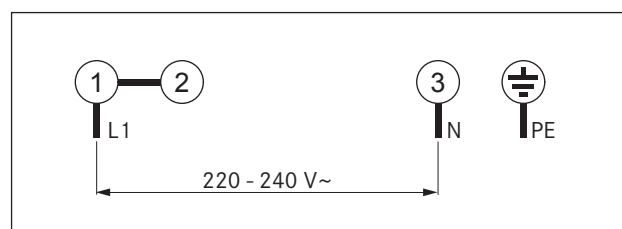
Fig. 5.23 Koblingsskjema 1-fase
