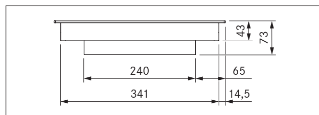
Fig. 3.3 PKCH2 apparatmål visning forfra
