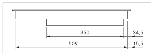
Fig. 3.4 PKCH2 apparatmål visning fra siden
