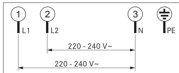
Fig. 5.22 Koblingsskjema 2-fase
