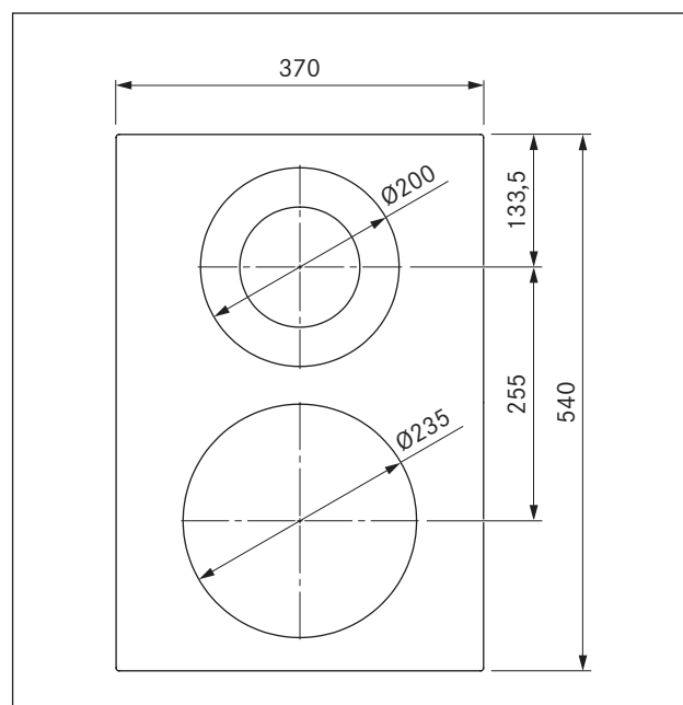
Fig. 3.2 PKCH2 apparatmål visning ovenfra
