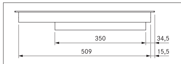
Afb. 3.4 PKCH2 Toestelafmetingen zijaanzicht
