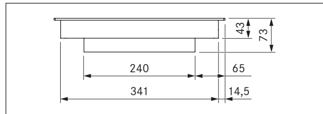
Afb. 3.3 PKCH2 Toestelafmetingen vooraanzicht
