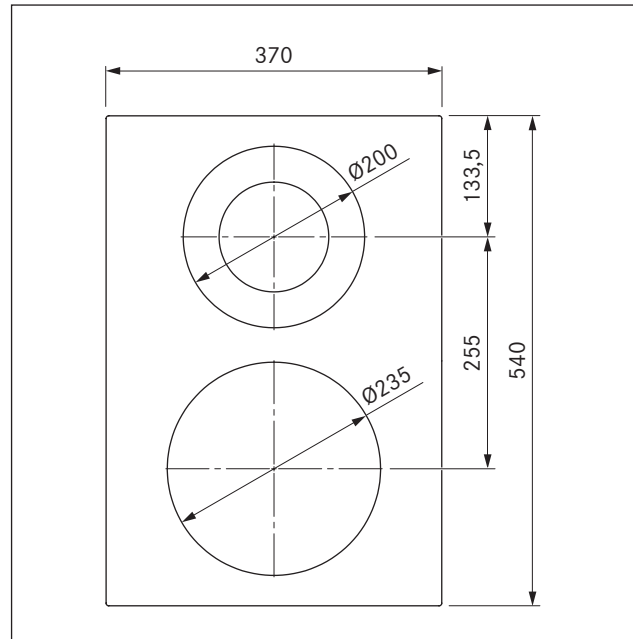
Afb. 3.2 PKCH2 Toestelafmetingen bovenaanzicht
