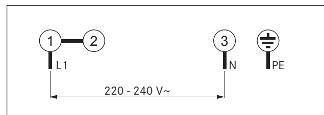
Afb. 5.23 Aansluitschema 1-fasig
