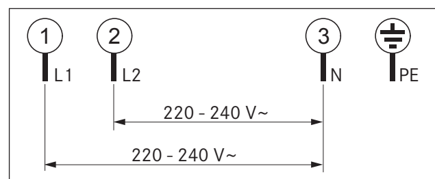
Afb. 5.22 Aansluitschema 2-fasig
