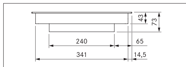
Afb. 3.3 PKCH2 Toestelafmetingen vooraanzicht
