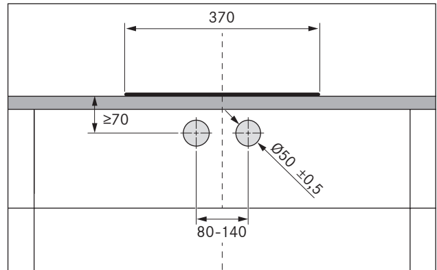
Kuva 5.8 Porauskuva
