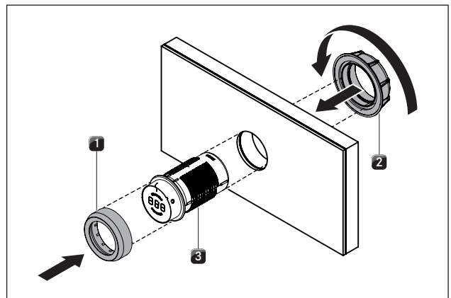
Kuva 5.9 Säätimen asentaminen
