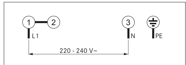
Kuva 5.23 Liitäntäkaavio – 1-vaiheinen liitäntä
