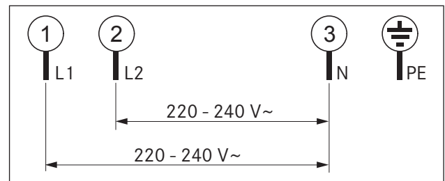
Kuva 5.22 Liitäntäkaavio – 2-vaiheinen liitäntä
