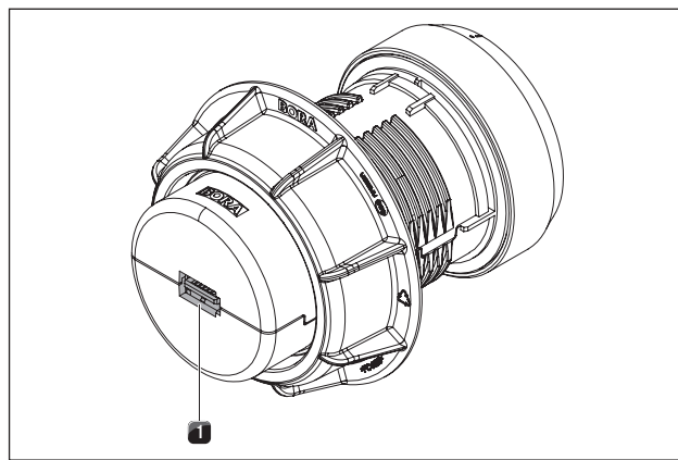
Fig. 5.18 Conexión mandos selectores lado posterior
