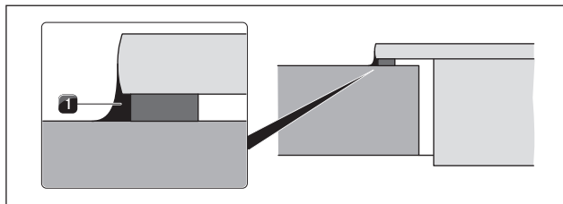
Fig. 5.17 Sellador de silicona en superposición
