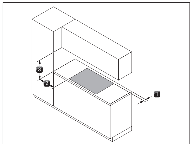
Fig. 5.15 Distancias mínimas con montaje girado 180°
