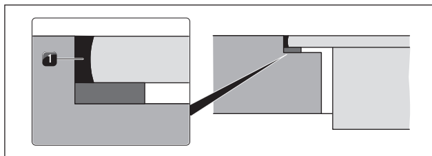
Fig. 5.16 Sellador de silicona en montaje enrasado
