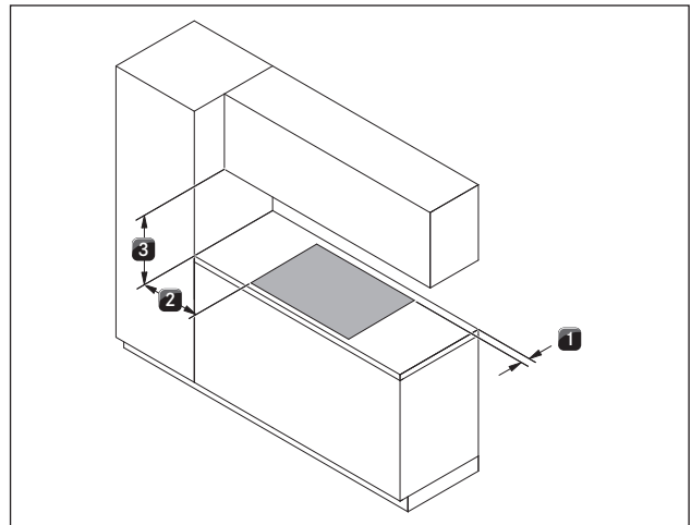
Fig. 5.15 Distancias mínimas con un montaje girado 180°
