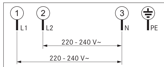
Fig. 5.22 Esquema de conexión bifásica
