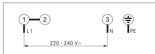
Fig. 5.23 Esquema de conexión monofásica
