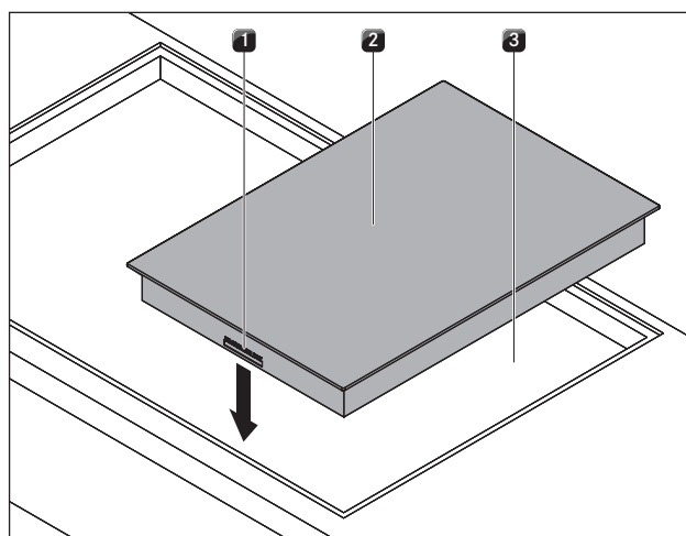
Fig. 5.12 Colocación de la placa de cocción
