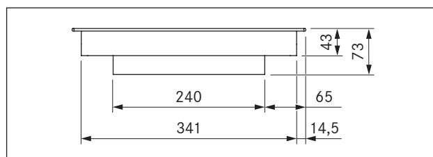
Fig. 3.3 PKCH2 dimensiones del aparato vista frontal
