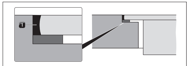
Fig. 5.16 Silicona de sellado para montaje enrasado
