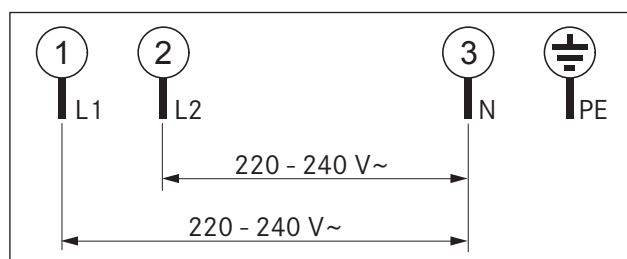
Fig. 5.22 Tilslutningsskema, 2-faset
