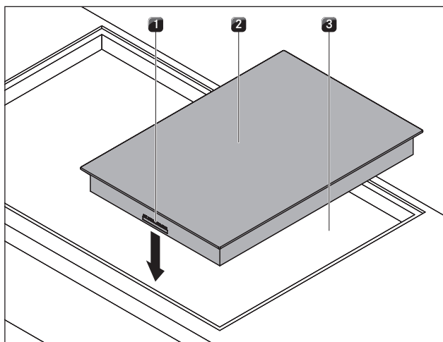
Sl. 5.14 Vstavitev kuhalne plošče
