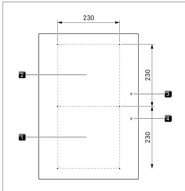
Fig. 3.8 Estrutura da placa de cozinhar PKFI3 e tamanho das zonas de cozedura
