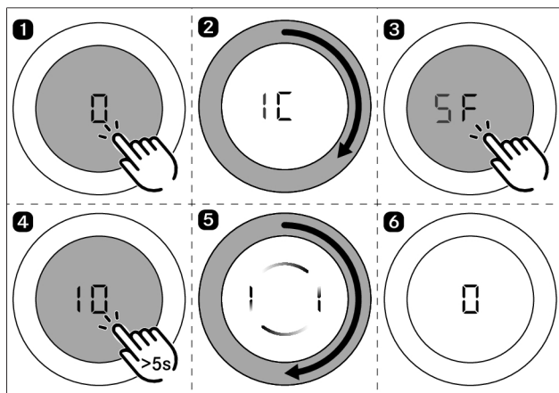
Fig. 5.21 Repor antecipadamente a vida útil do filtro
