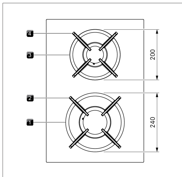
Fig. 3.15 Estrutura da placa de cozinhar a gás PKG3 e tamanho das zonas de cozedura
