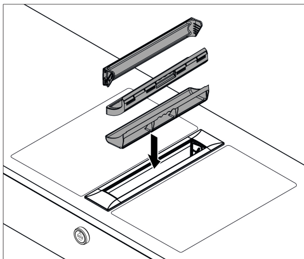
Fig. 7.2 Instalação dos componentes
