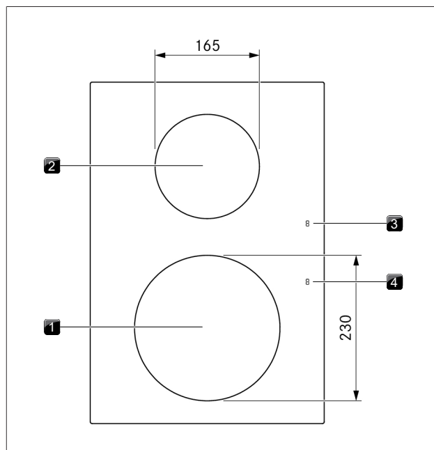
Fig. 3.9 Estrutura da placa de cozinhar PKI3 e tamanho das zonas de cozedura
