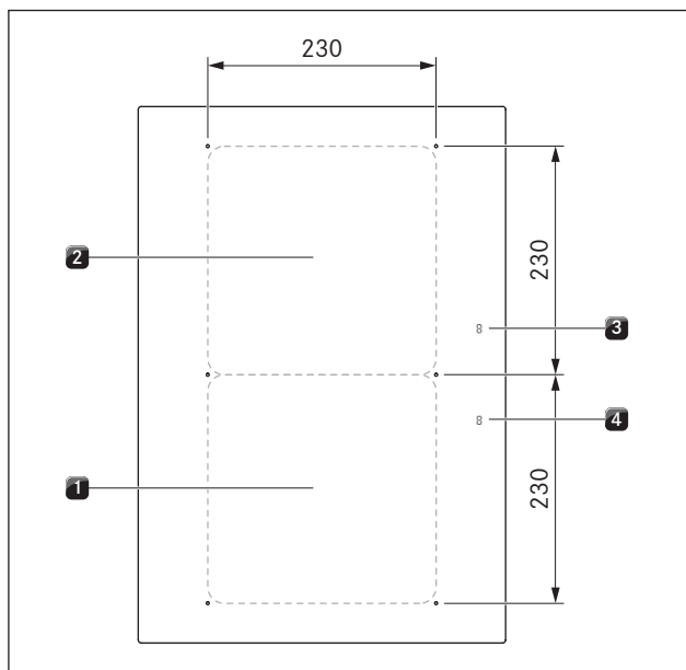
איור 4.8 מבנה הכיריים PKF13 וגודל אזורי הבישול
