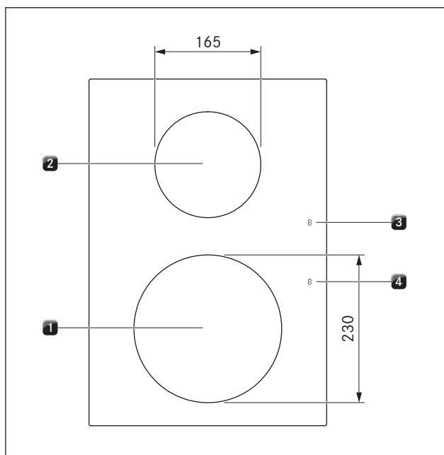
איור 4.9 מבנה הכיריים PKI3 וגודל אזורי הבישול
