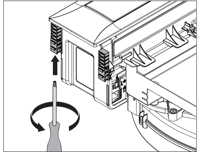
Kuva 4.31 Kiinnittimien kiristäminen
