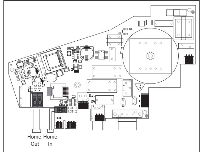
Kuva 4.45 Ulkoisten kytkinten liitäntäkaavio, PKAS3/PKAS3AB
