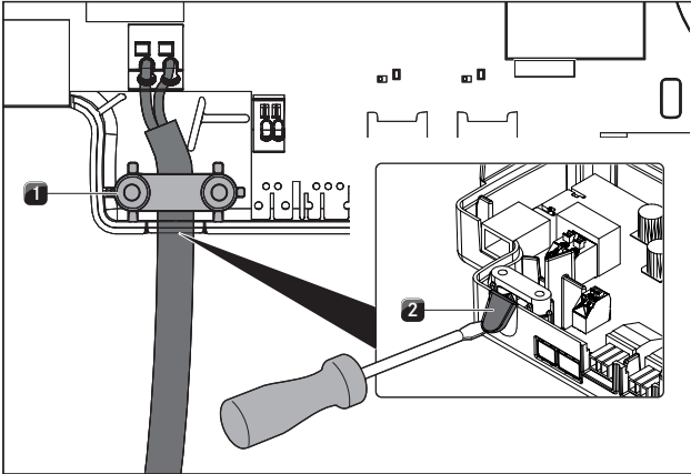
Kuva 4.47 Home out-liitännän teko ja vedonpoistin
