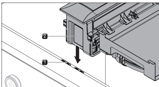
Kuva 4.26 Korkeussäätölevyt
