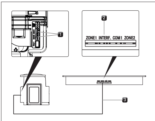
Kuva 4.55 Keittotason höyrynpoiston ja keittotasojen välisen tiedonsiirron muodostaminen
