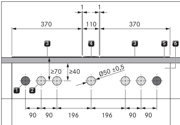
Kuva 4.13 Porauskuva: porausaukot kahdelle keittotasolle, yhdelle keittotason höyrynpoistolle ja kahdelle pistorasialle
