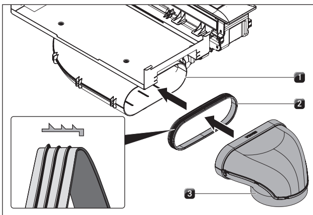
Kuva 4.36 Liittäminen kanavajärjestelmään
