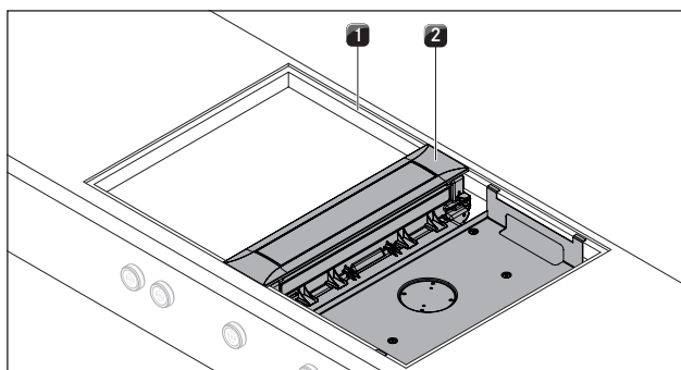
Kuva 4.25 Keittotason höyrynpoiston sovittaminen
