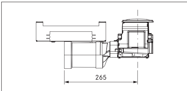
Kuva 4.34 Kanavaliitosmitat PKA3/PKA3AB ja suora kanavaosa
