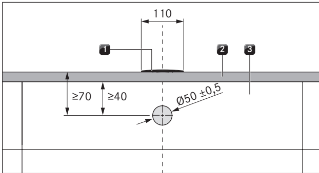
Kuva 4.12 Keittotason höyrynpoiston aukon porauskuva
