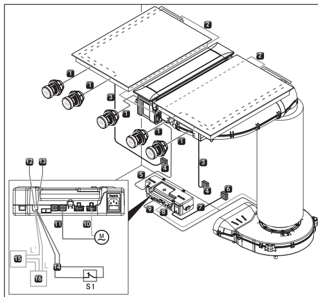
Kuva 4.56 Liitäntäkaavio PKA3/PKA3AB
