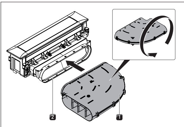
Kuva 4.21 Käyrän kanavaosan kääntäminen
