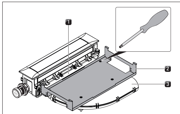
Kuva 4.18 Kannatinlevyn poistaminen
