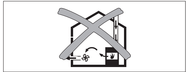
Kuva 4.1 Poistoilma-asennus – kielletty toteutus
