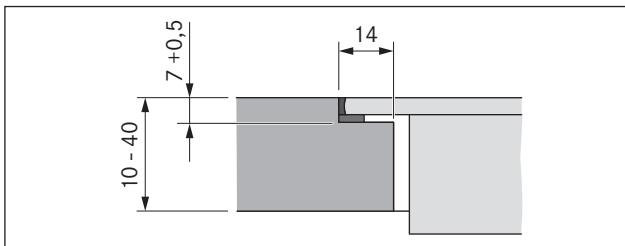
Kuva 4.8 Saumamitta uppoasennusta varten
