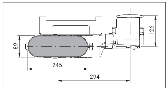
Kuva 4.32 Kanavaliitosmitat PKA3/PKA3AB ja käyrä kanavaosa
