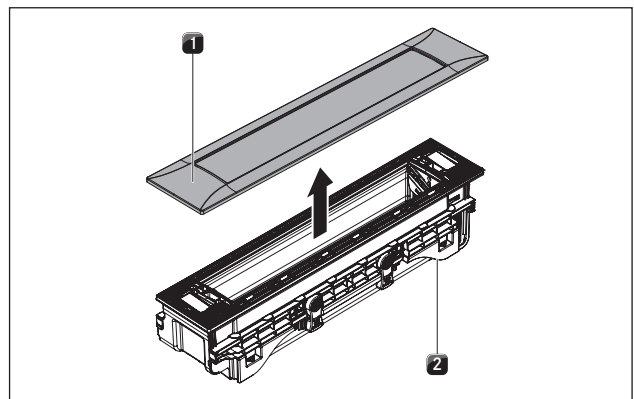
Kuva 4.24 Peitekehysten irrottaminen
