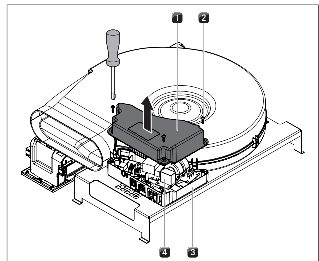
Kuva 4.39 Ohjausyksikön kotelon kannen avaaminen
