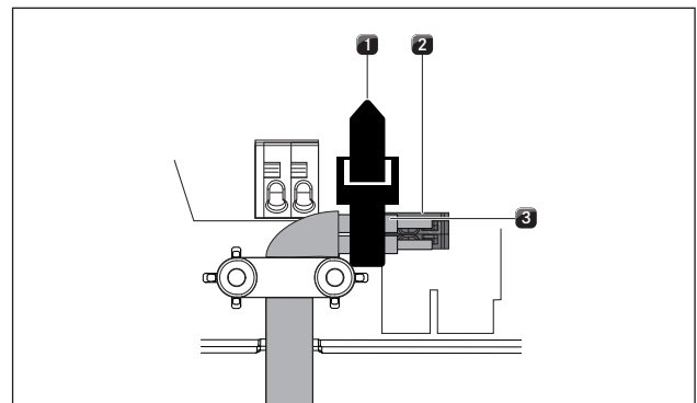
Kuva 4.46 Home in -liitännän johtoside PKAS3/PKAS3AB
