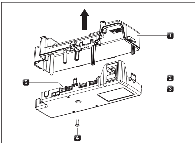
Kuva 4.40 Ohjausyksikön kotelon kannen avaaminen
