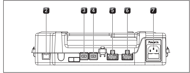
Kuva 4.53 Ohjausyksikön liitännät
