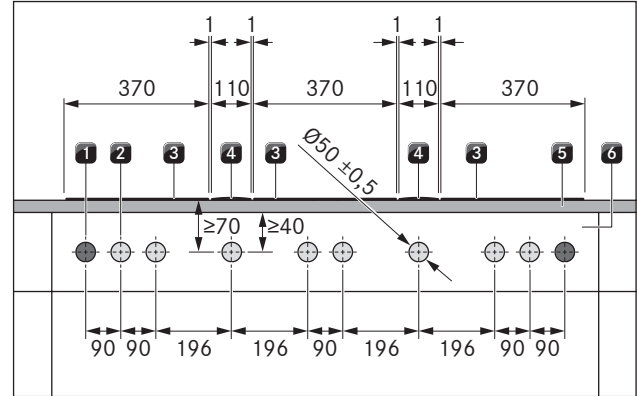
Kuva 4.14 Porauskuva: porausaukot kolmelle keittotasolle, kahdelle keittotason höyrynpoistolle ja kahdelle pistorasialle
