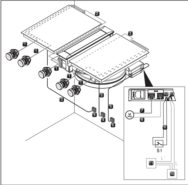
Kuva 4.57 Liitäntäkaavio PKAS3/PKAS3AB
