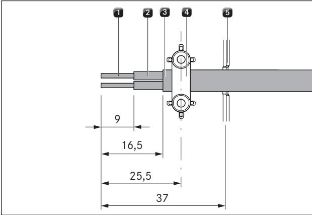
Kuva 4.43 Liitäntäjohdon kuorintapituudet ja asennusasento, PKAS3/PKAS3AB – home out
