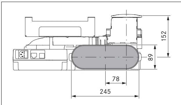
Kuva 4.35 Kanavaliitosmitat PKAS3, PKAS3AB
