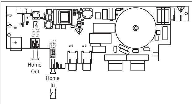
Kuva 4.44 Ulkoisten kytkinten liitäntäkaavio, PKA3/PKA3AB
