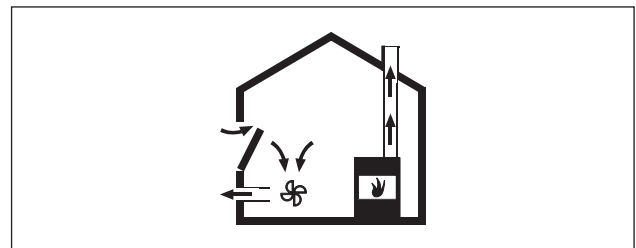
Kuva 4.2 Poistoilma-asennus – oikea toteutus
