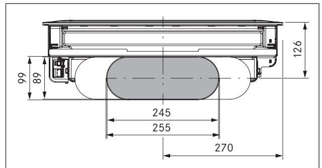
Kuva 4.33 Kanavaliitosmitat PKA3/PKA3AB ja suora kanavaosa
