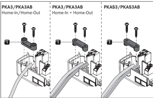
Kuva 4.48 Vedonpoistimen asennus
