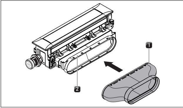
Kuva 4.20 Suoran kanavaosan asentaminen
