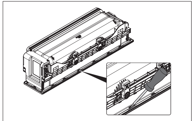
Kuva 4.23 Peitekehysten irrottaminen
