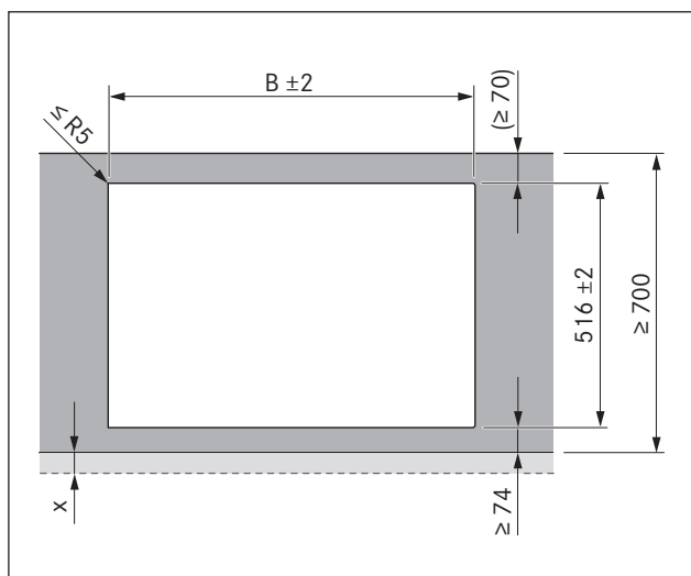
Kuva 4.9 Asennusaukkojen mitat pinta-asennusta varten
