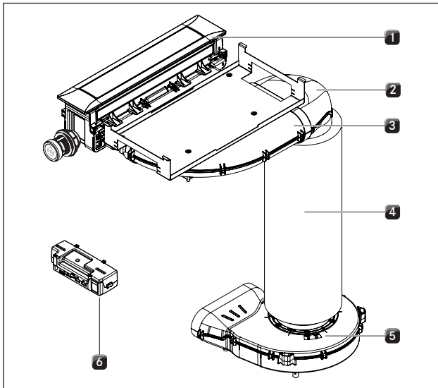
Kuva 4.38 Vakioasennus PKA3/PKA3AB
