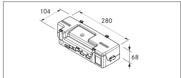
Kuva 3.4 Ohjauksyksikön laitemitat
