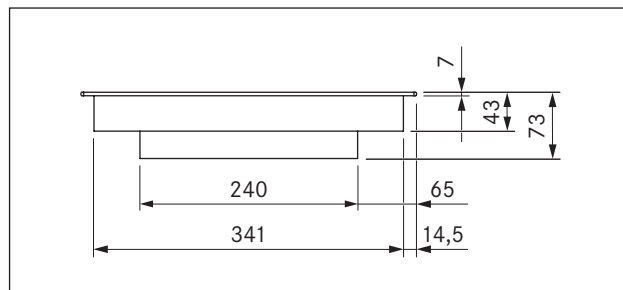
рис. 3.5 Размеры РКСЗВ: вид спереди
