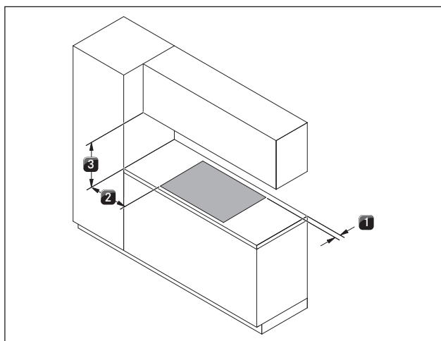
Fig. 5.15 Distância mínima da instalação a 180°
