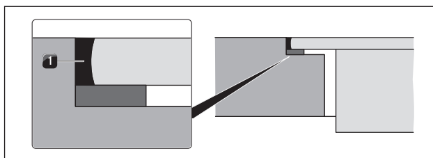
Fig. 5.16 Massa vedante de silicone na montagem à face
