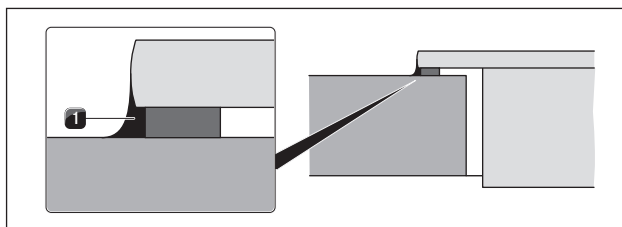
Fig. 5.17 Massa vedante de silicone na montagem por sobreposição
