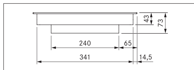
Fig. 3.2 PKC32 dimensões do aparelho vista frontal
