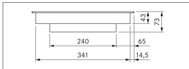
Fig. 3.5 PKC3B dimensões do aparelho vista frontal
