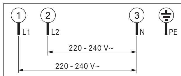
Fig. 5.22 Esquema de ligação bifásica
