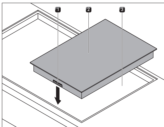
Fig. 5.14 Insert cooktop
