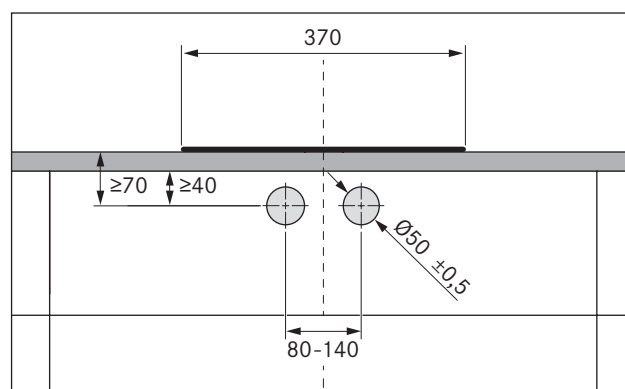
Fig. 5.8 Drill template
