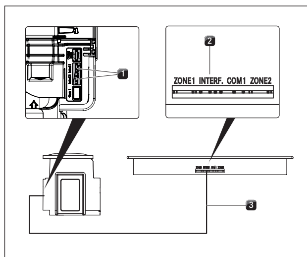
Obr. 5.22 Připojka automatického odtahu
