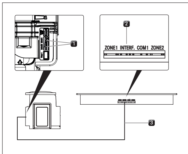
Fig. 5.22 Connecteur du système d'aspiration automatique
