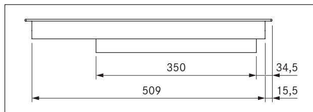
Fig. 3.6 Dimensions PKC3B vue de côté
