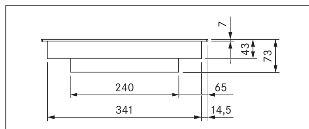
Fig. 3.5 Dimensions PKC3B vue de face
