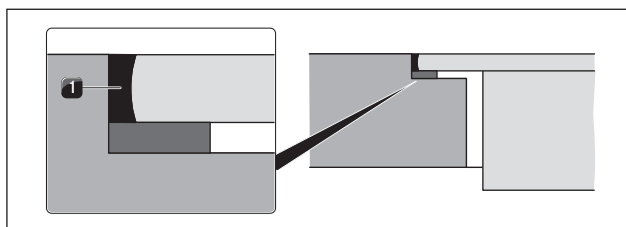
Fig. 5.25 Joint en silicone en montage affleurant
