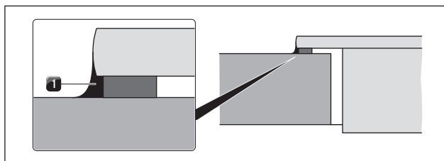
Fig. 5.26 Joint en silicone en montage en saillie
