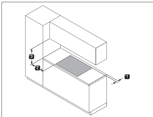
Fig. 5.17 Distances minimales en montage à 180°
