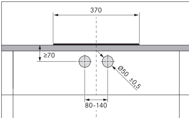
bild 5.9 Borrbild
