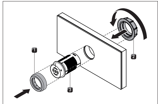
bild 5.12 Vridknapp monterad
