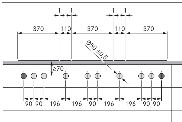
bild 5.14 Borrhål vid 3 spishällar och 2 ångsugar
