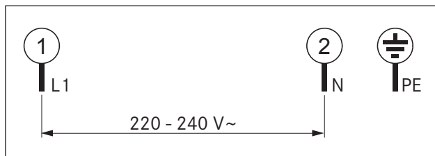
bild 5.22 Anslutningsschema 1-fasigt
