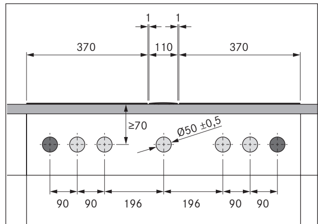
bild 5.13 Borrhål vid 2 spishällar och 1 ångsug
