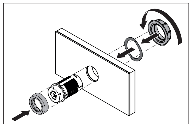
Obr. 5.13 Montáž ovládacieho kolieska
