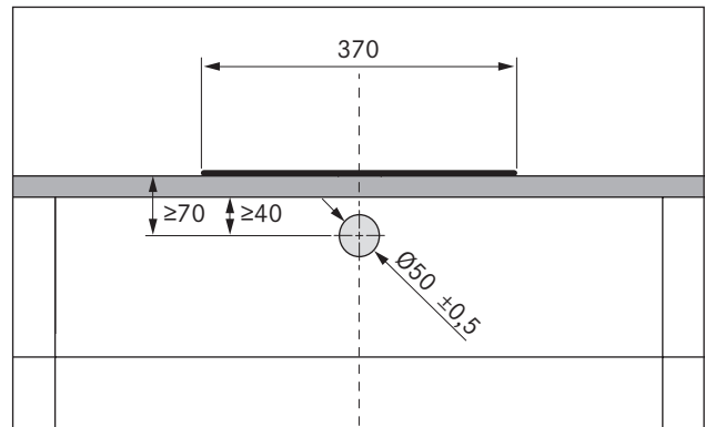
Obr. 5.11 Vrtacia šablóna
