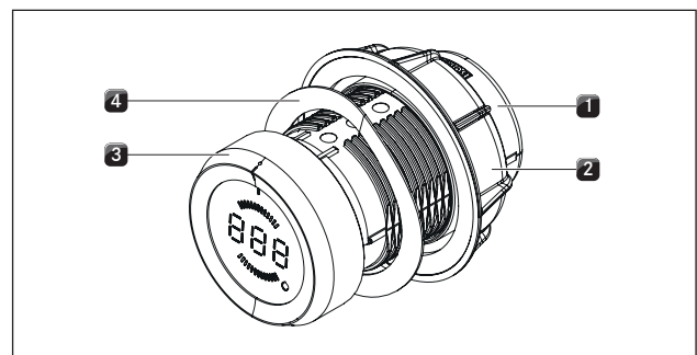
Obr. 5.12 Konštrukcia ovládacieho kolieska
