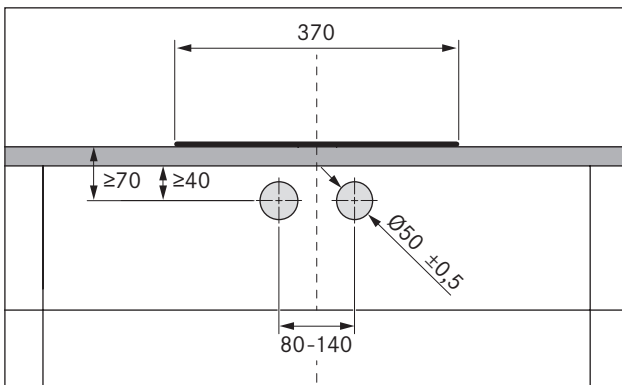
Obr. 5.9 Vrtacia šablóna
