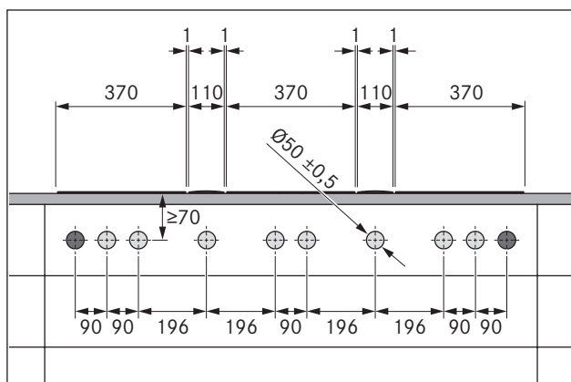
Fig. 5.14 Perfuração do painel para 3 placas de cozinha e 2 exaustores de placa
