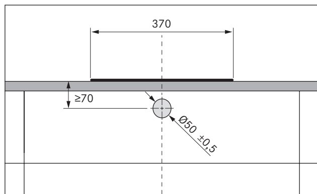
Fig. 5.11 Diagrama de perfuração
