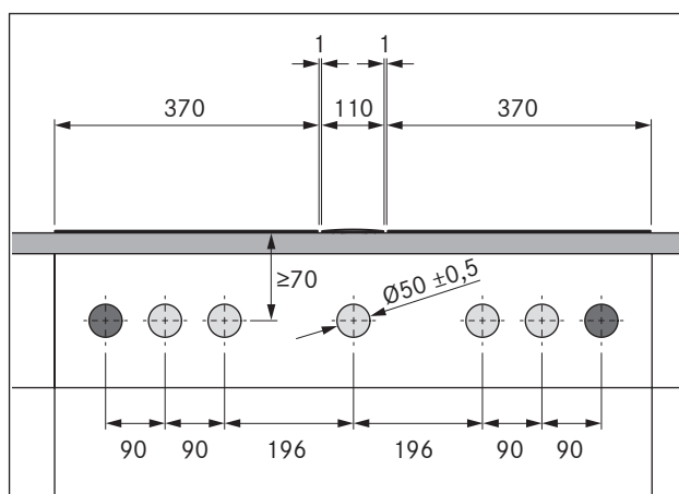
Fig. 5.13 Perfuração do painel para 2 placas de cozinhar e 1 exaustor de placa
