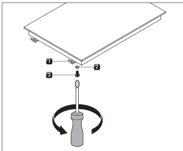
Ilustracja 5.19 Klamry mocujące
