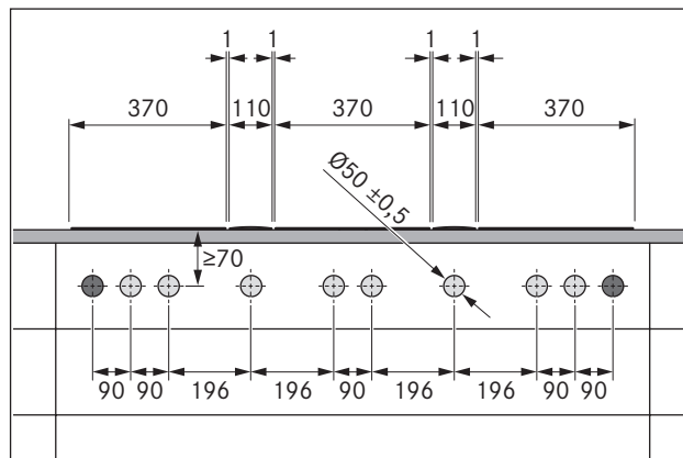
Afb. 5.14 Boorgaten in het paneel bij 3 kookvelden en 2 afzuigingen
