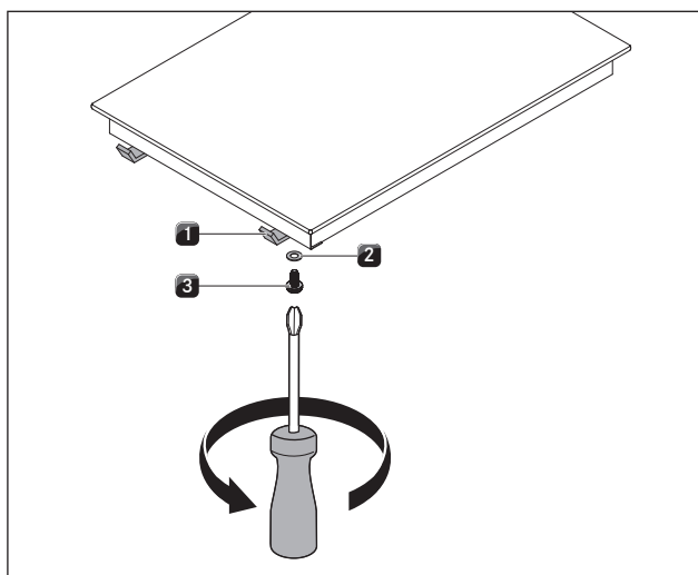
Afb. 5.17 Bevestigingsklemmen
