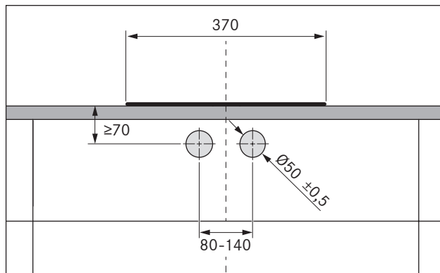
Afb. 5.9 Boorpatroon
