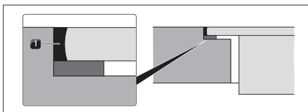
Afb. 5.18 Siliconenkit bij vlakbouw
