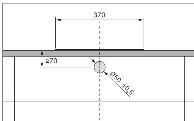
Afb. 5.11 Boorpatroon
