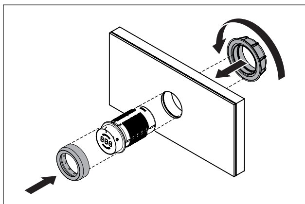
Afb. 5.12 Bedieningsknop monteren
