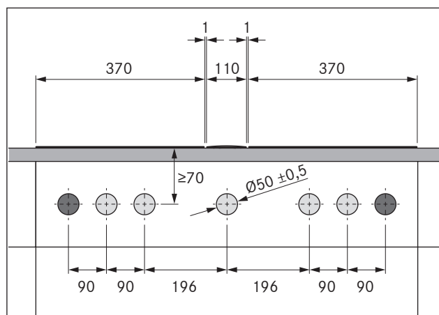
Afb. 5.13 Boorgaten in het paneel bij 2 kookvelden en 1 afzuiging
