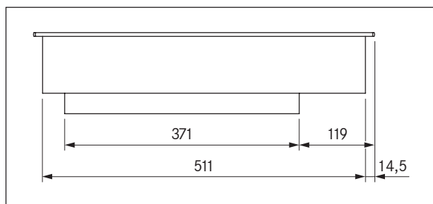
Afb. 3.4 PKIW1 Toestelafmetingen zijaanzicht
