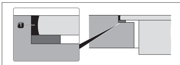
Afb. 5.18 Siliconenkit bij vlainbouw
