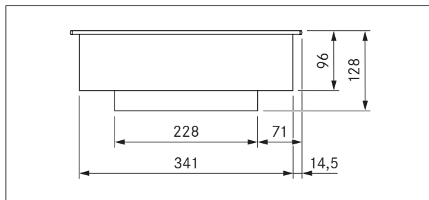
Afb. 3.3 PKIW1 Toestelafmetingen vooraanzicht
