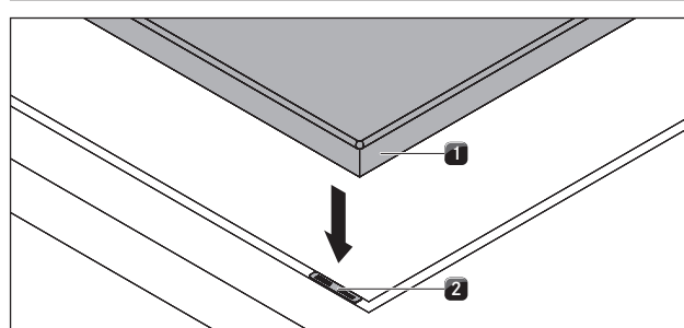
Afb. 5.16 Kookveld en vulplaatjes
