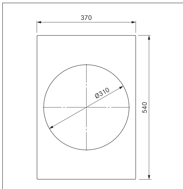
Afb. 3.2 PKIW1 Toestelafmetingen bovenaanzicht
