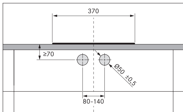
Afb. 5.9 Boorpatroon
