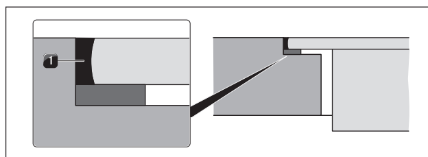
Fig. 5.18 Sigillante in silicone per montaggio a filo piano
