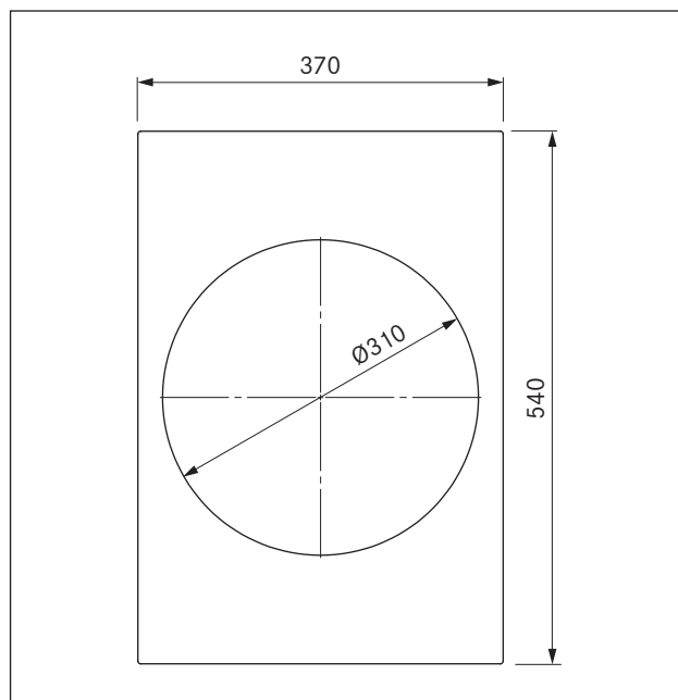
Fig. 3.2 PKIW1 Dimensioni apparecchio vista da sopra
