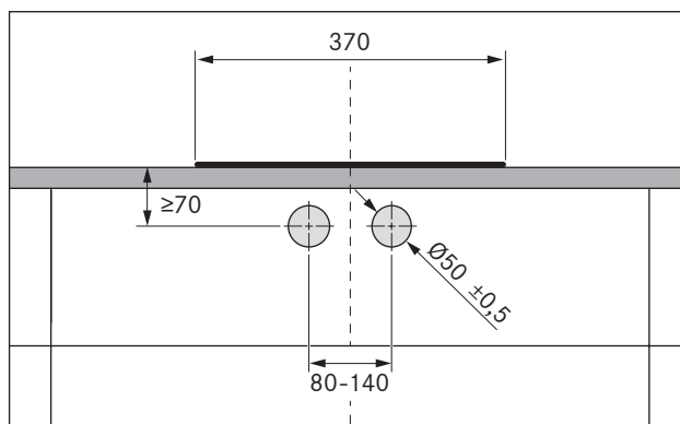
Fig. 5.9 Schema di foratura
