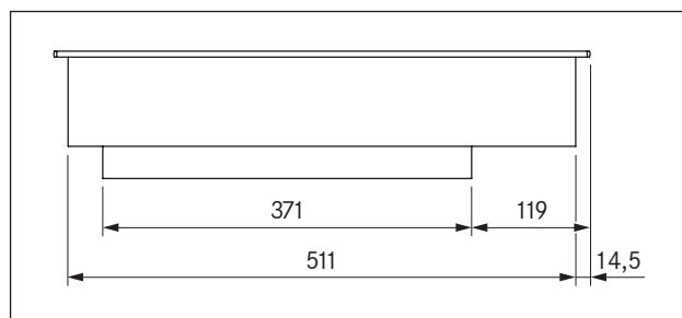
Fig. 3.4 PKIW1 Dimensioni apparecchio vista laterale
