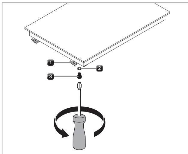
Fig. 5.17 Staffe di fissaggio
