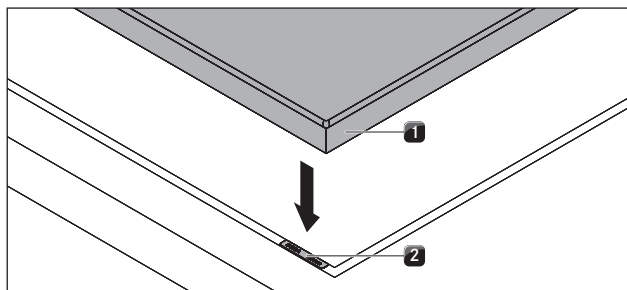
Fig. 5.16 Piano cottura e pannelli di compensazione altezza
