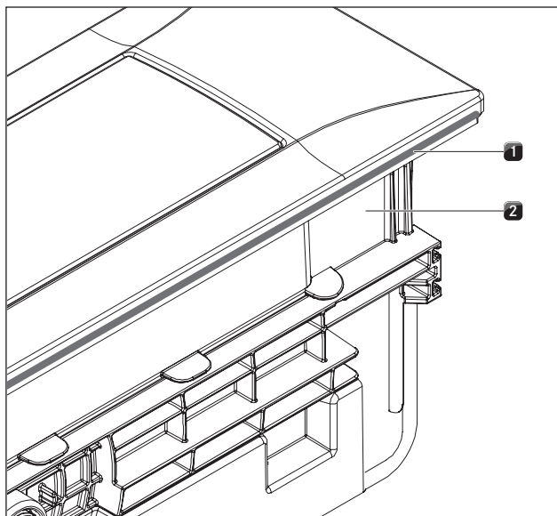
Fig. 5.7 Rimuovere la cornicetta laterale in plastica dell'aspiratore per piano cottura
