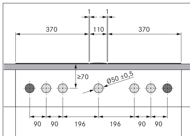
Fig. 5.13 Forature per pannelli di copertura con 2 piani cottura e 1 aspiratore
