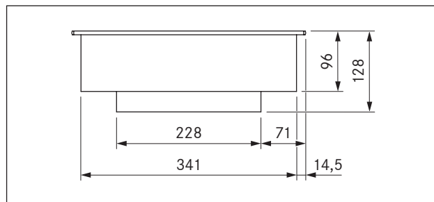
Fig. 3.3 PKIW1 Dimensioni apparecchio vista anteriore
