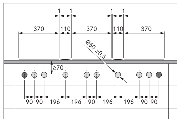
Fig. 5.14 Forature pannello di copertura per 3 piani cottura e 2 aspiratori
