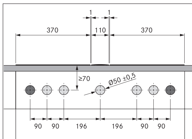
Fig. 5.13 Perçage de bandeau pour 2 tables de cuisson et 1 dispositif d'aspiration
