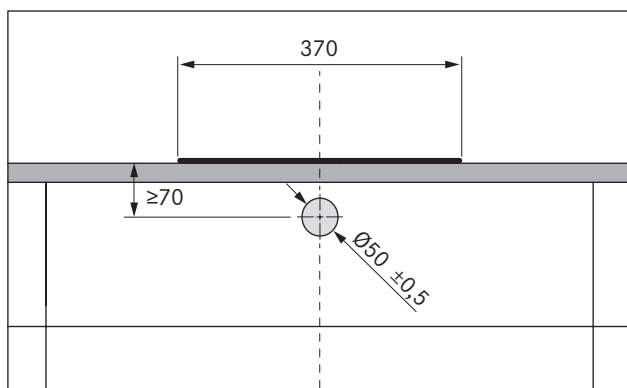
Fig. 5.11 Schéma de perçage
