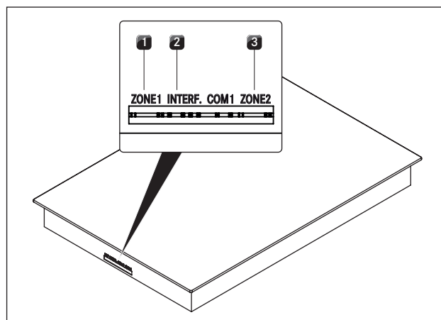
Fig. 5.21 Connecteurs de la table de cuisson
