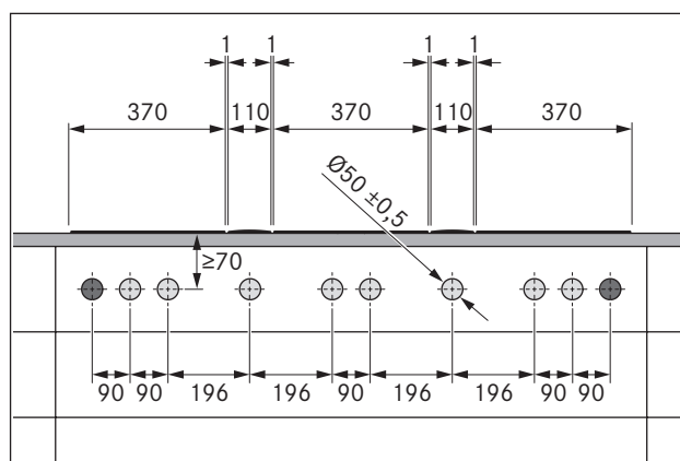
Fig. 5.14 Perçage de bandeau pour 3 tables de cuisson et 2 dispositifs d'aspiration
