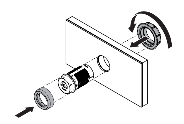
Fig. 5.12 Montez le bouton de commande
