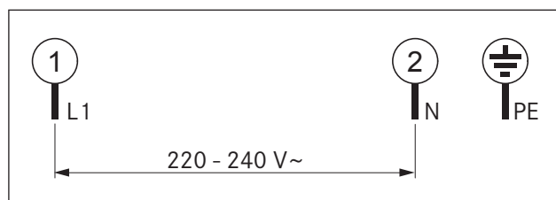
Fig. 5.22 Schéma de raccordement 1 phase
