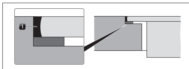
Fig. 5.18 Pâte de silicone pour montage affleurant
