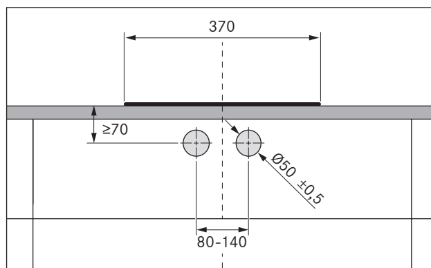
Fig. 5.9 Schéma de perçage
