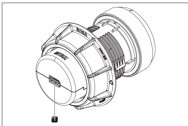
Fig. 5.20 Raccordement du bouton de commande sur la face arrière
