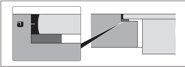
Sl. 5.24 Silikonska tesnilna masa pri montaži v isti ravni s površino
