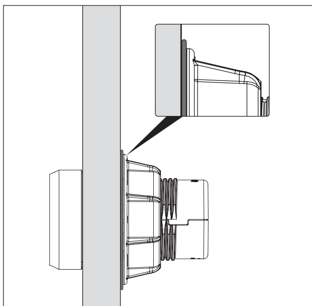
Sl. 5.14 Valovita vzmet po zaključeni montaži
