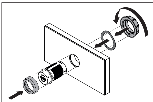
рис. 5.13 Установка поворотной ручки управления
