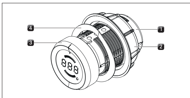
рис. 5.12 Конструкция поворотной ручки управления
