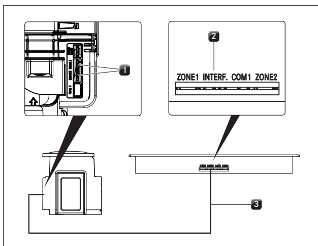
рис. 5.22 Соединение автоматики вытяжки
