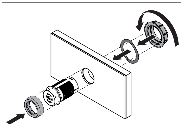
Afb. 5.13 Bedieningsknop monteren
