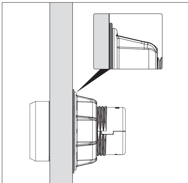
Afb. 5.14 Golfringveer na voltooide montage
