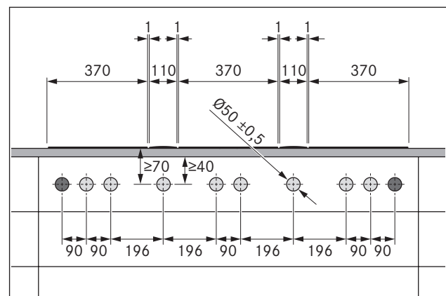
Fig. 5.16 Perforaciones en el frontal con 3 placas de cocción y 2 extractores de superficie
