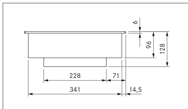
Fig. 3.3 PKIW1 dimensiones del aparato vista frontal
