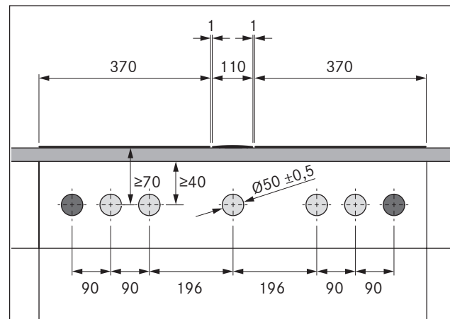
Fig. 5.15 Perforaciones en el frontal con 2 placas de cocción y 1 extractor de superficie
