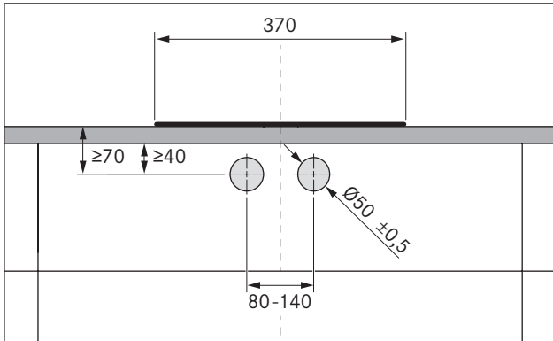
Fig. 5.9 Plantilla para taladrar
