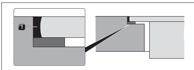
Fig. 5.24 Silicona de sellado para montaje enrasado
