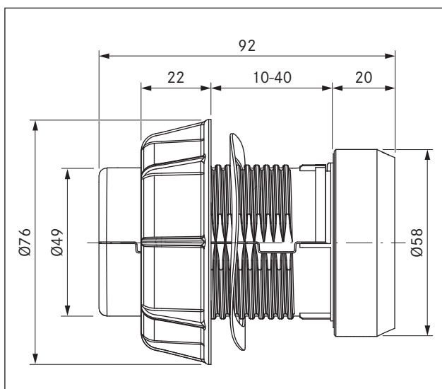
Fig. 3.1 Dimensiones del aparato mando selector
