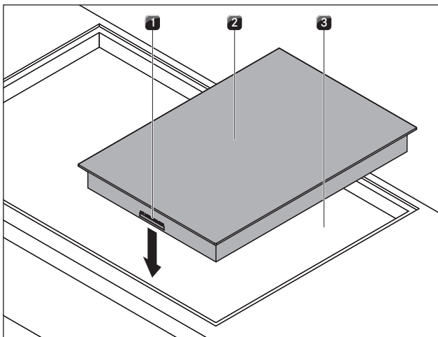
Fig. 5.17 Colocación de la placa de cocción
