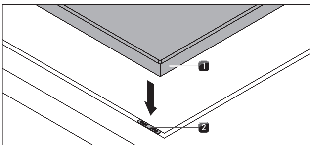
Fig. 5.18 Placa de cocción y placas de compensación de altura
