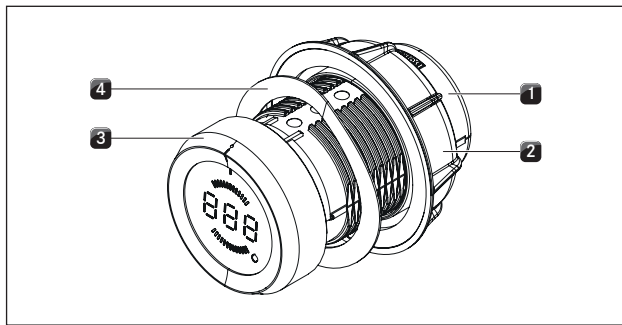
Fig. 5.12 Montaje mando selector
