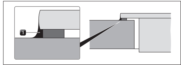
Fig. 5.25 Silicona de sellado para montaje superpuesto
