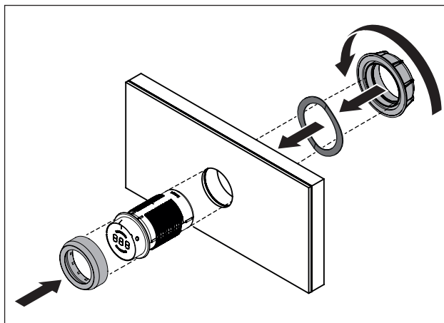
Fig. 5.13 Montar el mando selector
