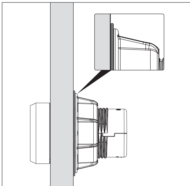
Fig. 5.14 Axselfjeder efter at monteringen er afsluttet
