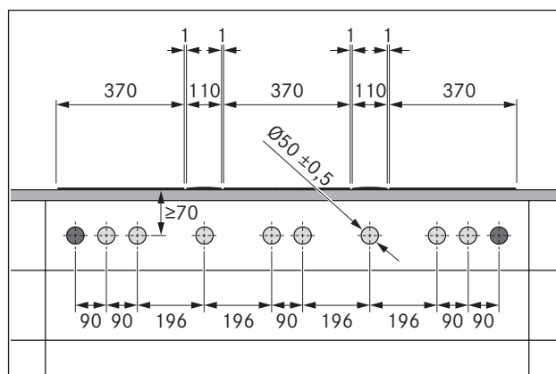
Fig. 5.11 Perfurações do painel em 3 placas de cozinhar e 2 extractores
