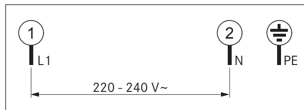
Fig. 5.21 Esquema de ligações, ligação monofásica
