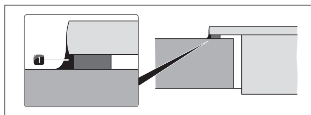
Afb. 5.16 Siliconenkit bij opbouwmontage
