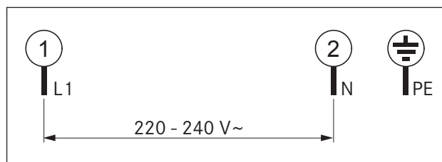
Afb. 5.21 Aansluitschema 1-fasig
