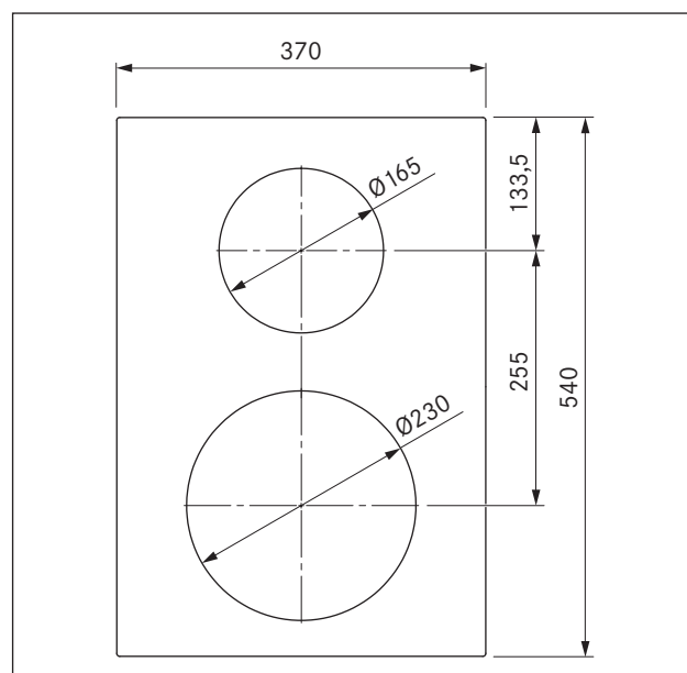
Afb. 3.2 PKI11 Toestelafmetingen bovenaanzicht
