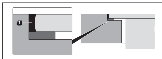
Afb. 5.15 Siliconenkit bij vlakinbouw
