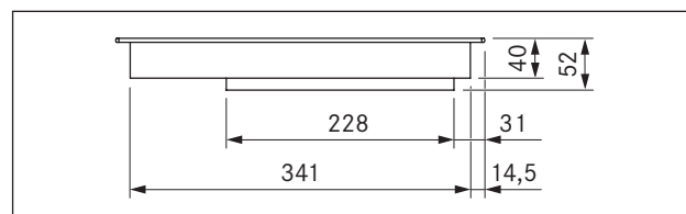
Afb. 3.3 PKI11 Toestelafmetingen vooraanzicht
