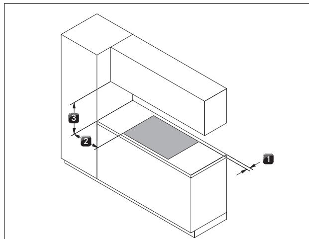
Fig. 5.1 Distanze minime
