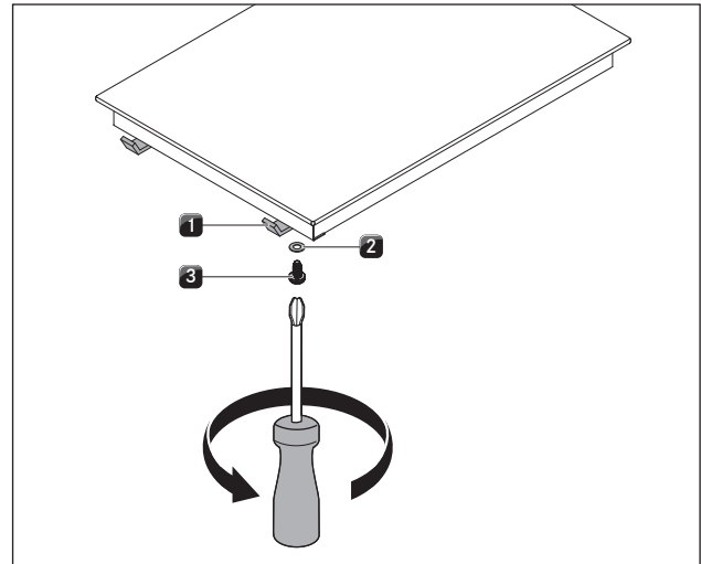
Fig. 5.14 Abrazaderas de montaje
