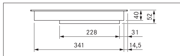
Fig. 3.3 PKI11 dimensiones del aparato vista frontal
