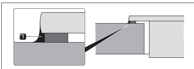
Fig. 5.16 Sellador de silicona en superposición
