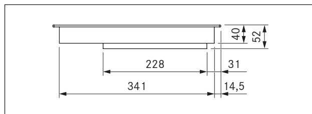
SI. 3.3 Dimenzije naprave PKFI11, pogled od spredaj
