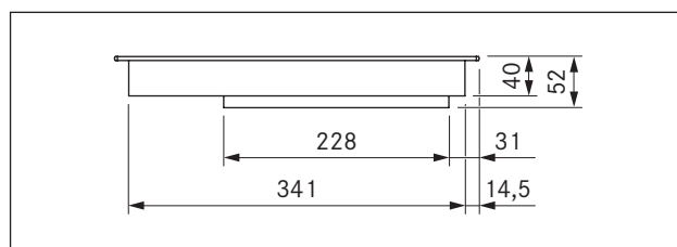
Fig. 3.3 PKFI11 dimensões do aparelho vista frontal
