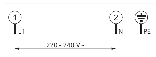
Fig. 5.21 Esquema de ligação monofásica
